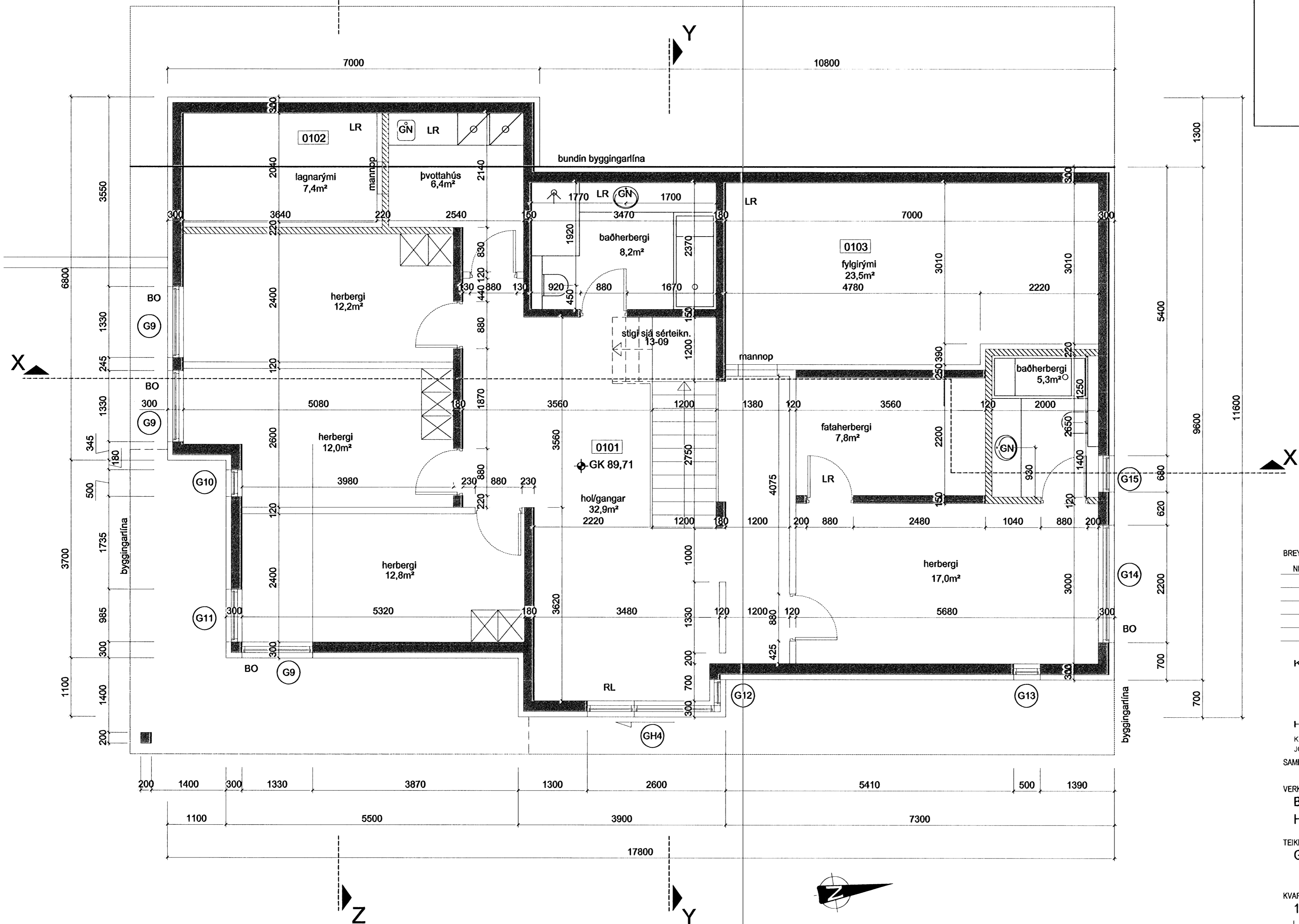
GRUNNMYND 1. HÆÐ 1:50
