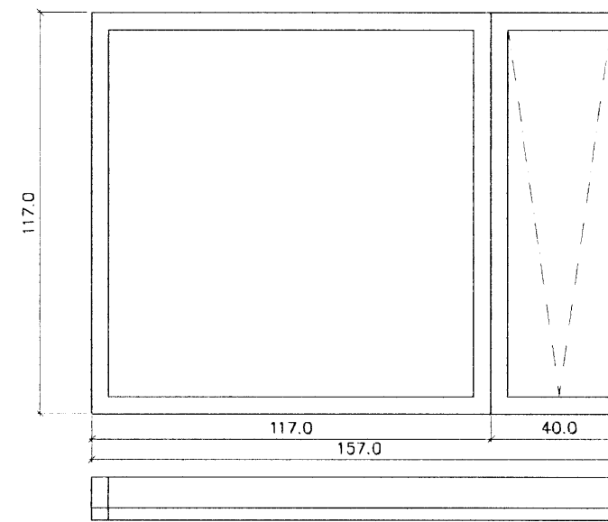
G3 1.stk. gluggi með opnanlegu fagi.
