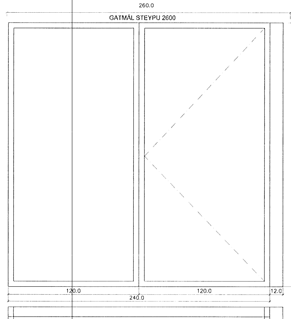
G6 1.stk. Horngluggi með rennihurð.
