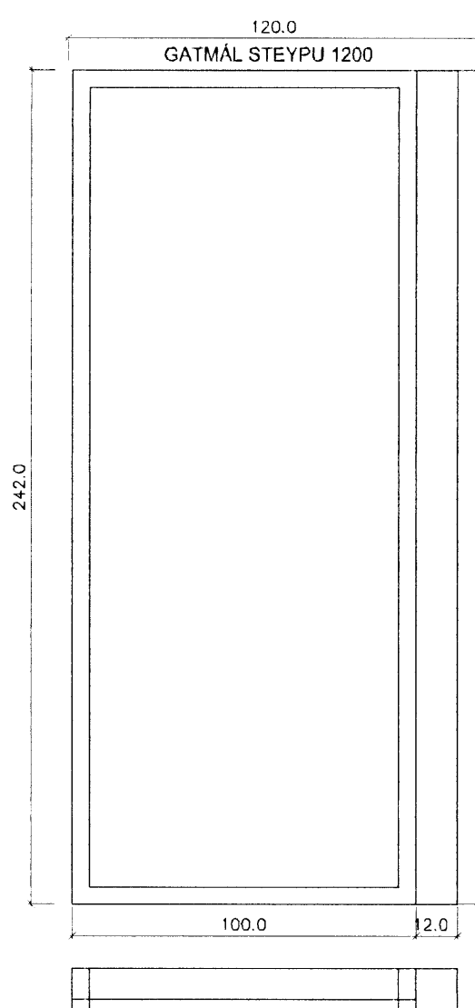
G5 1.stk. Horngluggi með rennihurð.
