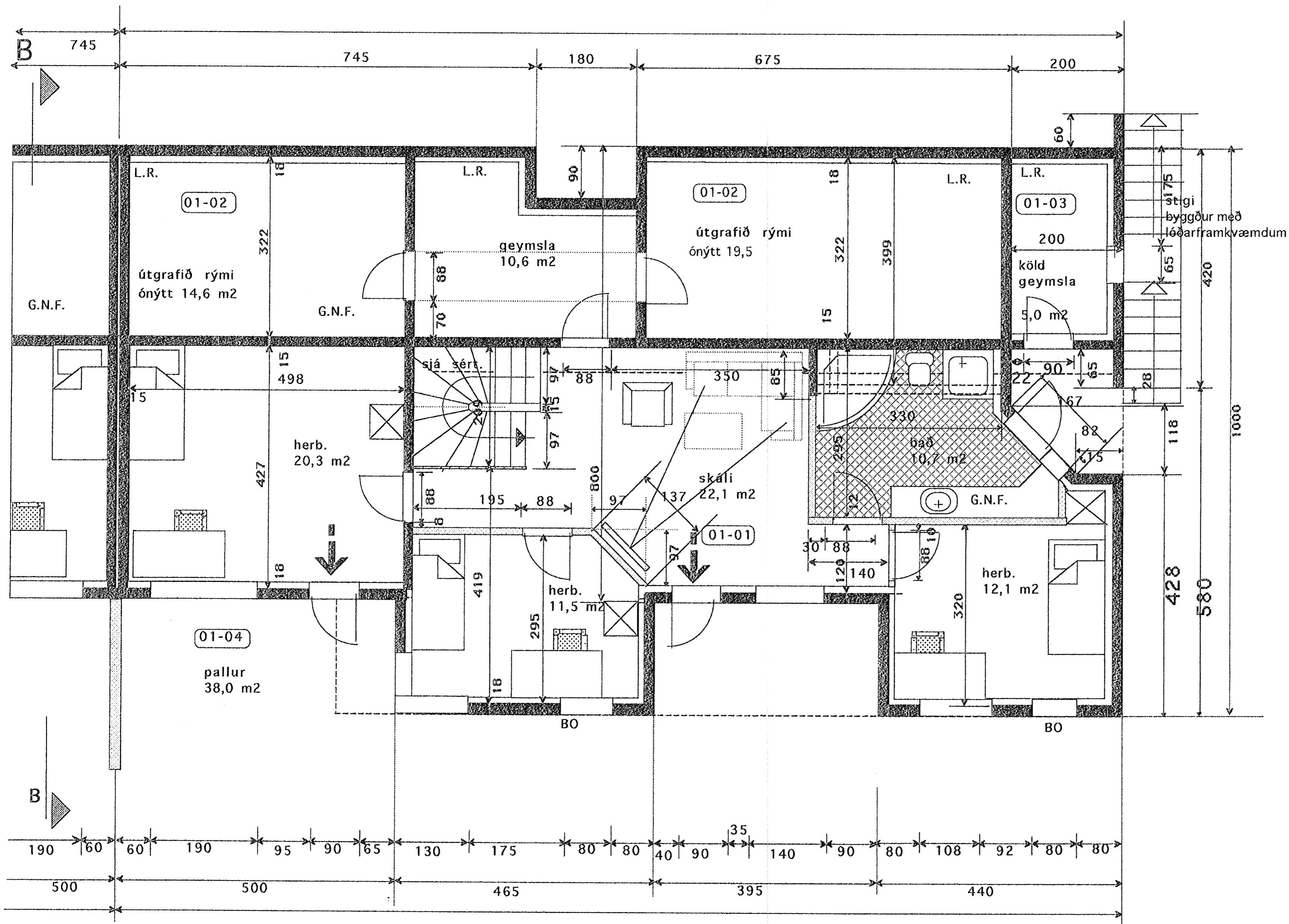
Grunnmynd 1. hæð 1:50
