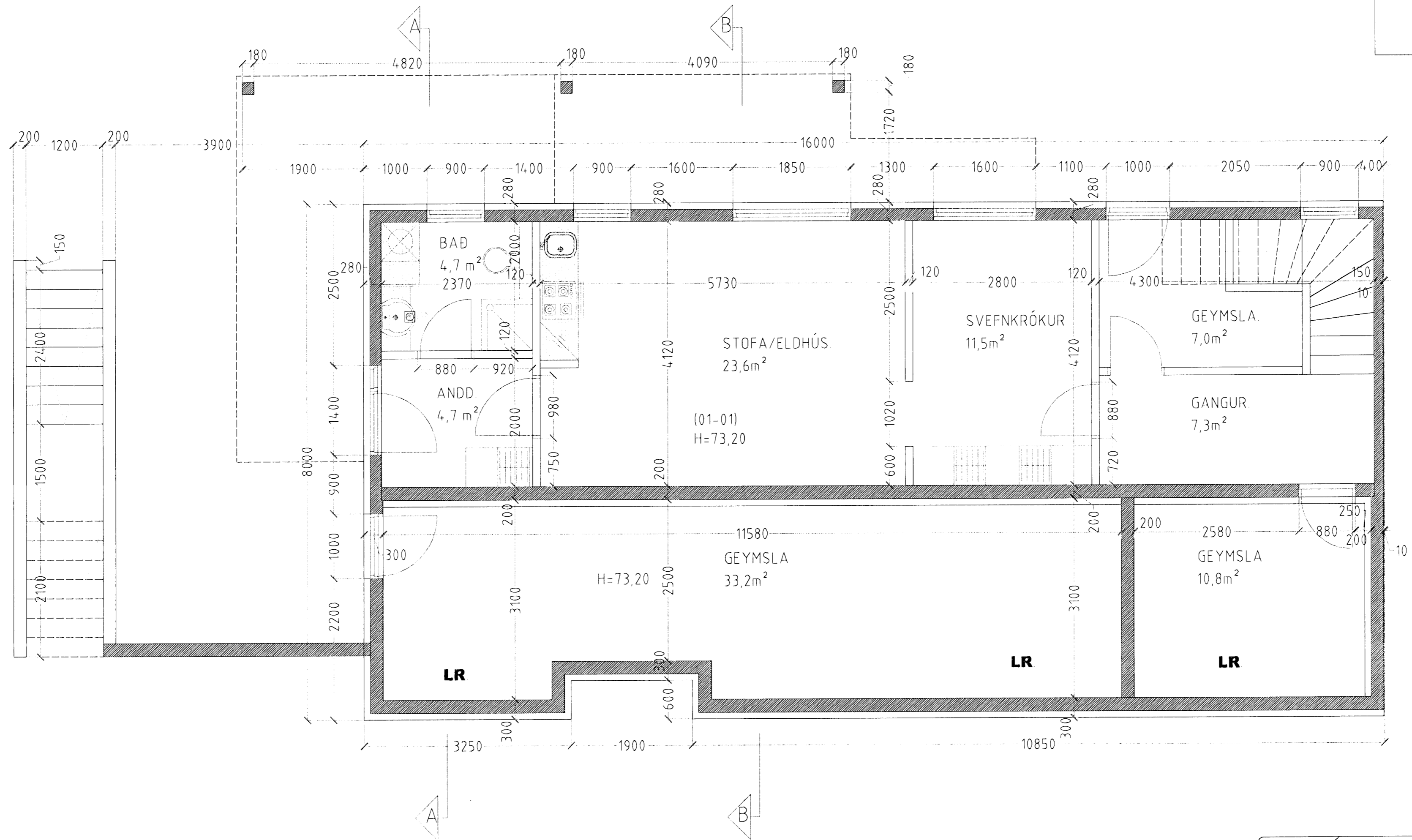
GRUNNMYND JARÐHÆÐ MKV. 1:50.
