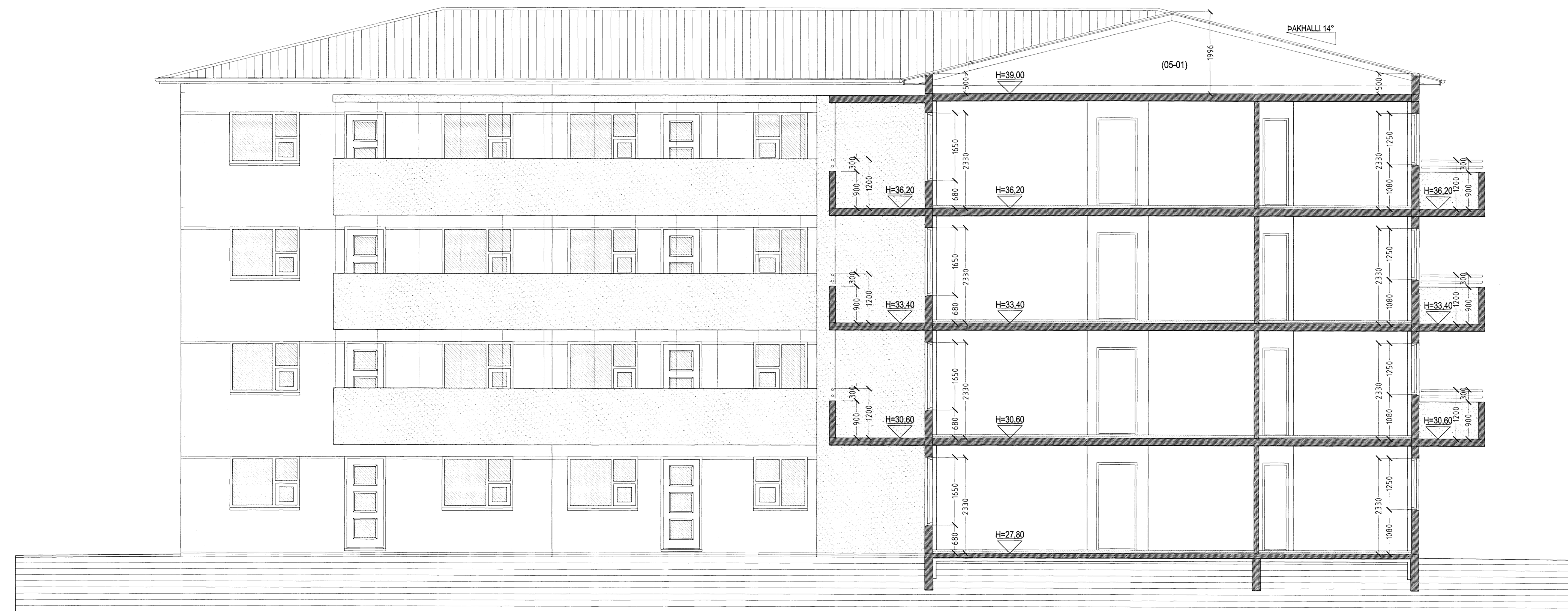
SNID C-C MKV. 1:50.
