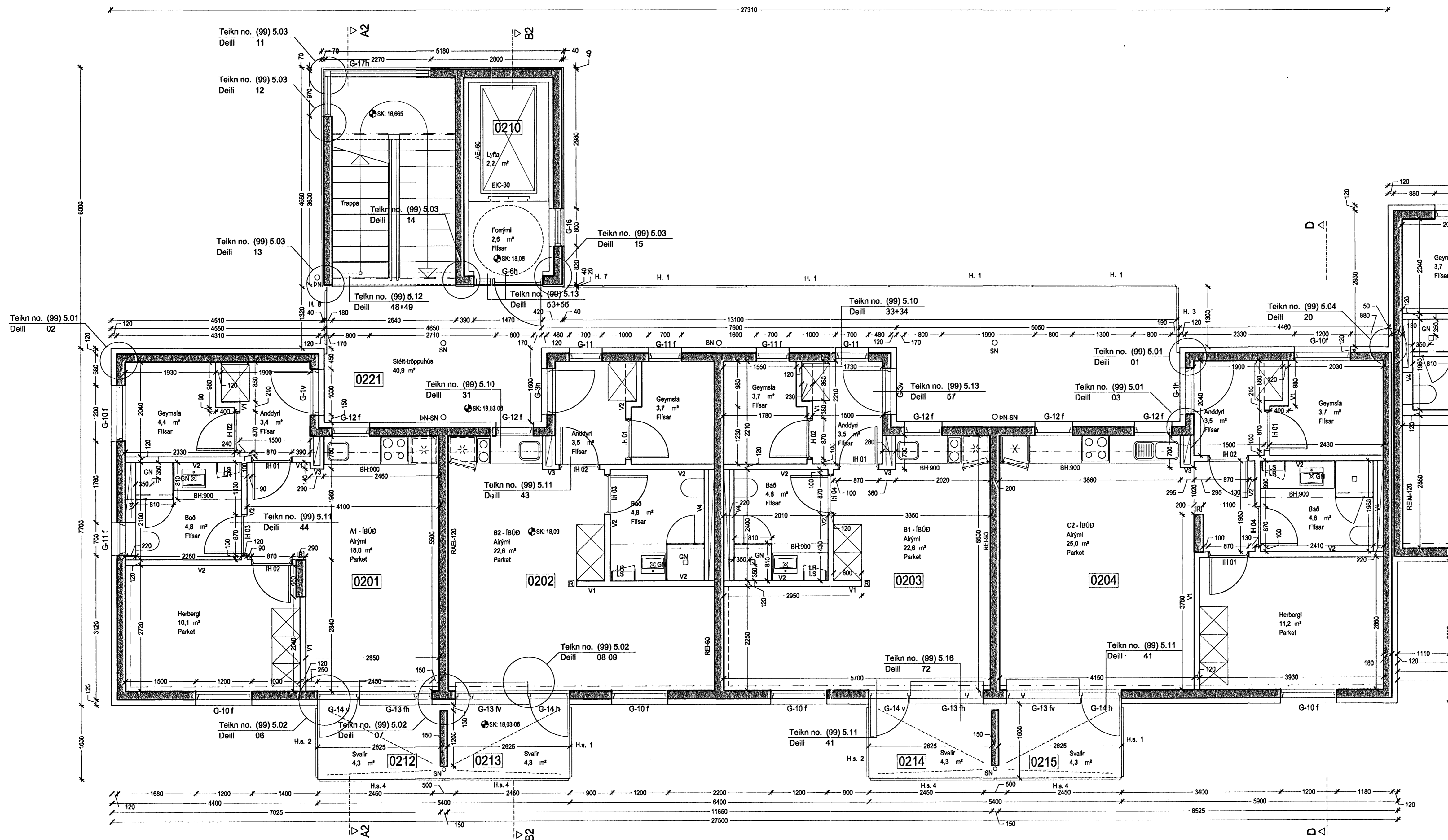
Grunnmynd 2.hæð, mkv. 1:50
