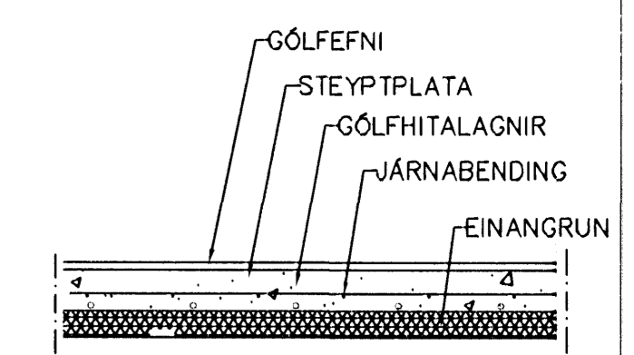
LAGNIR, SNIÐ, 1:20
