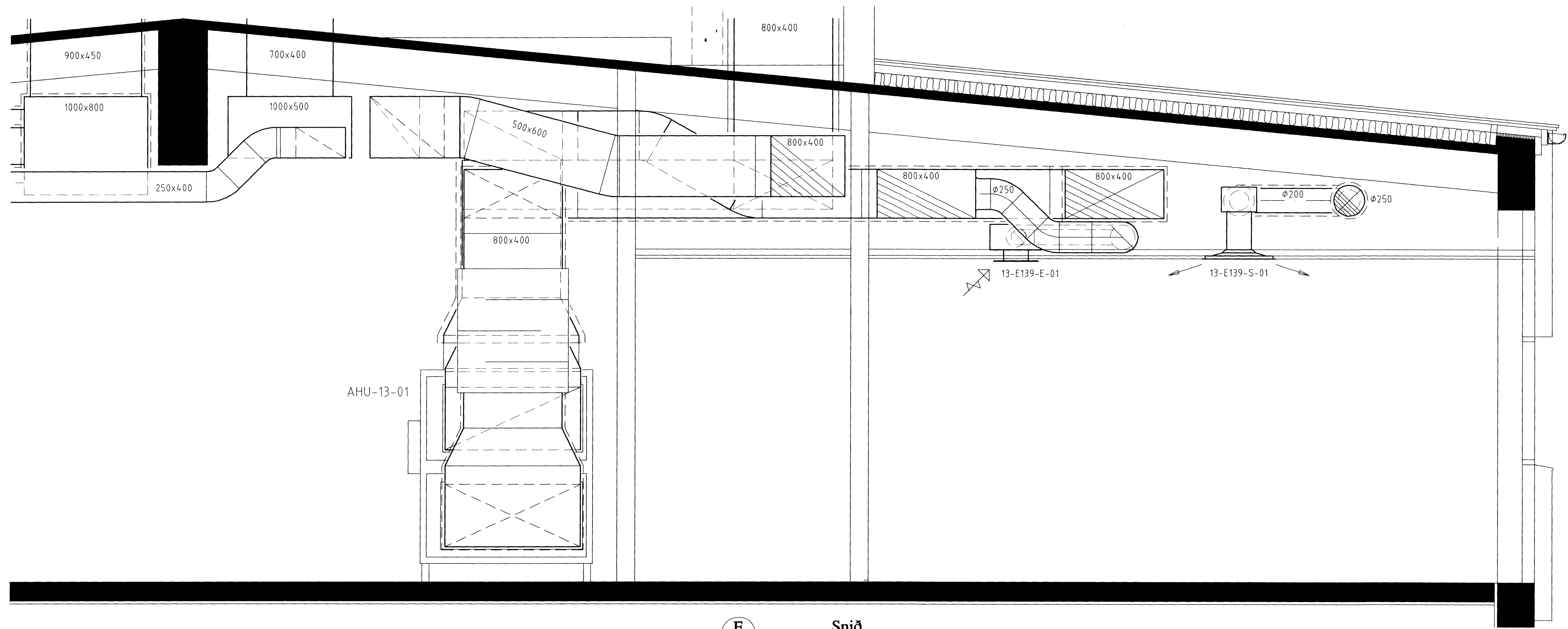
E 202304 Snið Mkv. 1: 20
