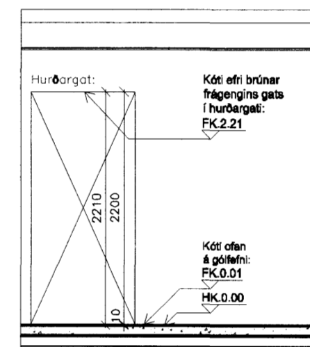
SNÍÐ 2, 1:50
