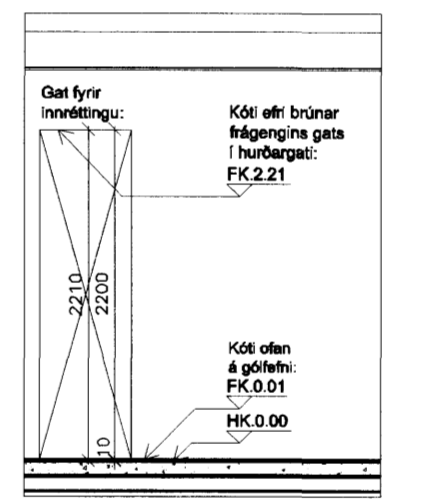
SNÍÐ 4, 1:50
