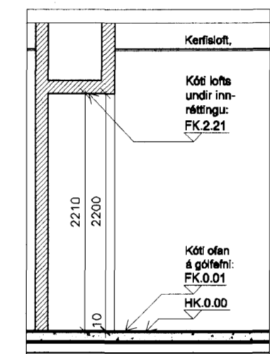
SNÍÐ 1, 1:50
