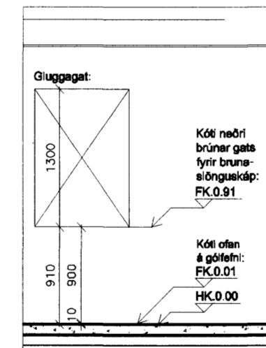
SNÍÐ 5, 1:50
