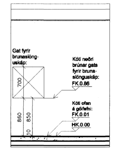
SNÍÐ 3, 1:50
