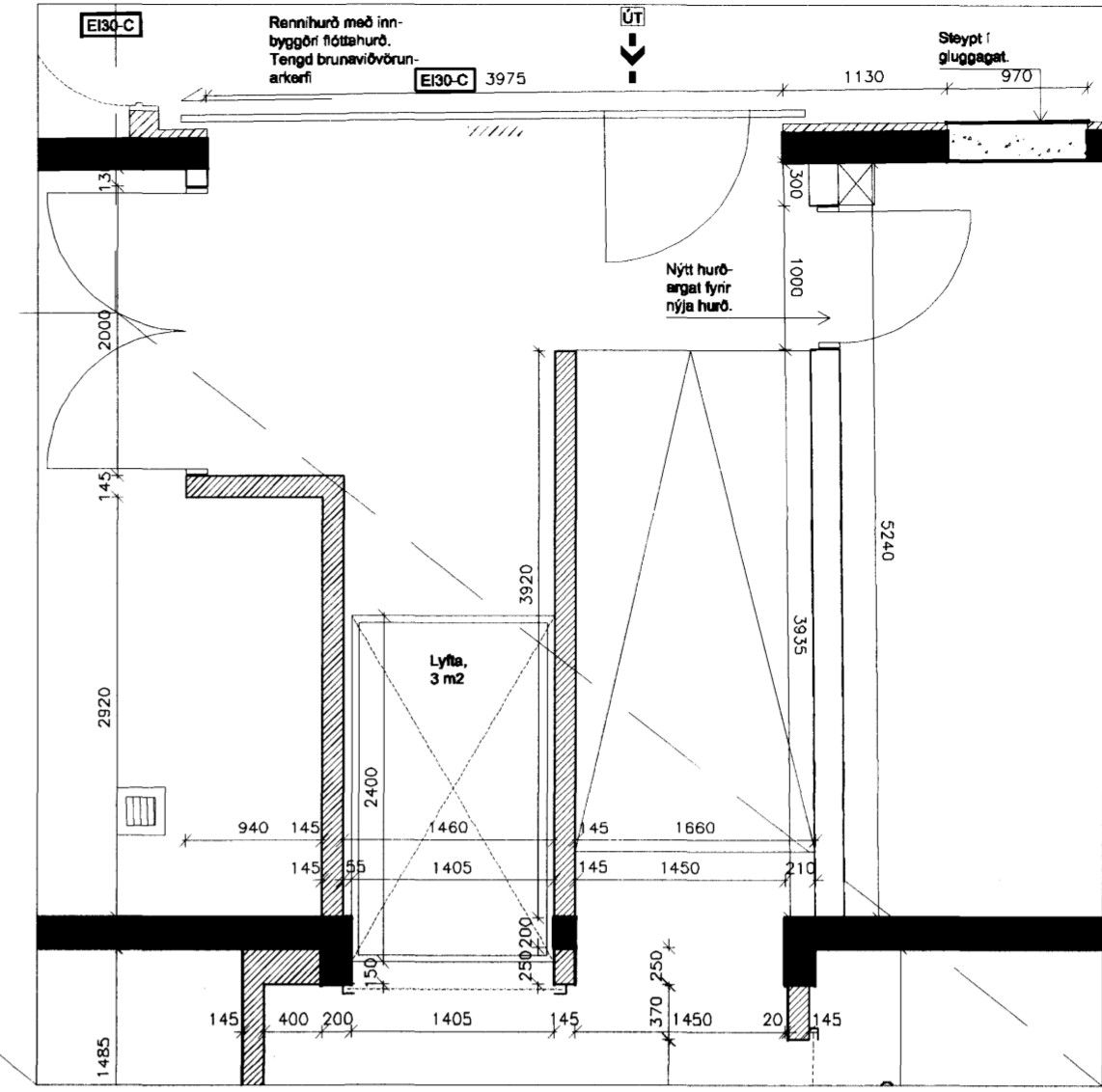
GRUNNMYND, 1:50
