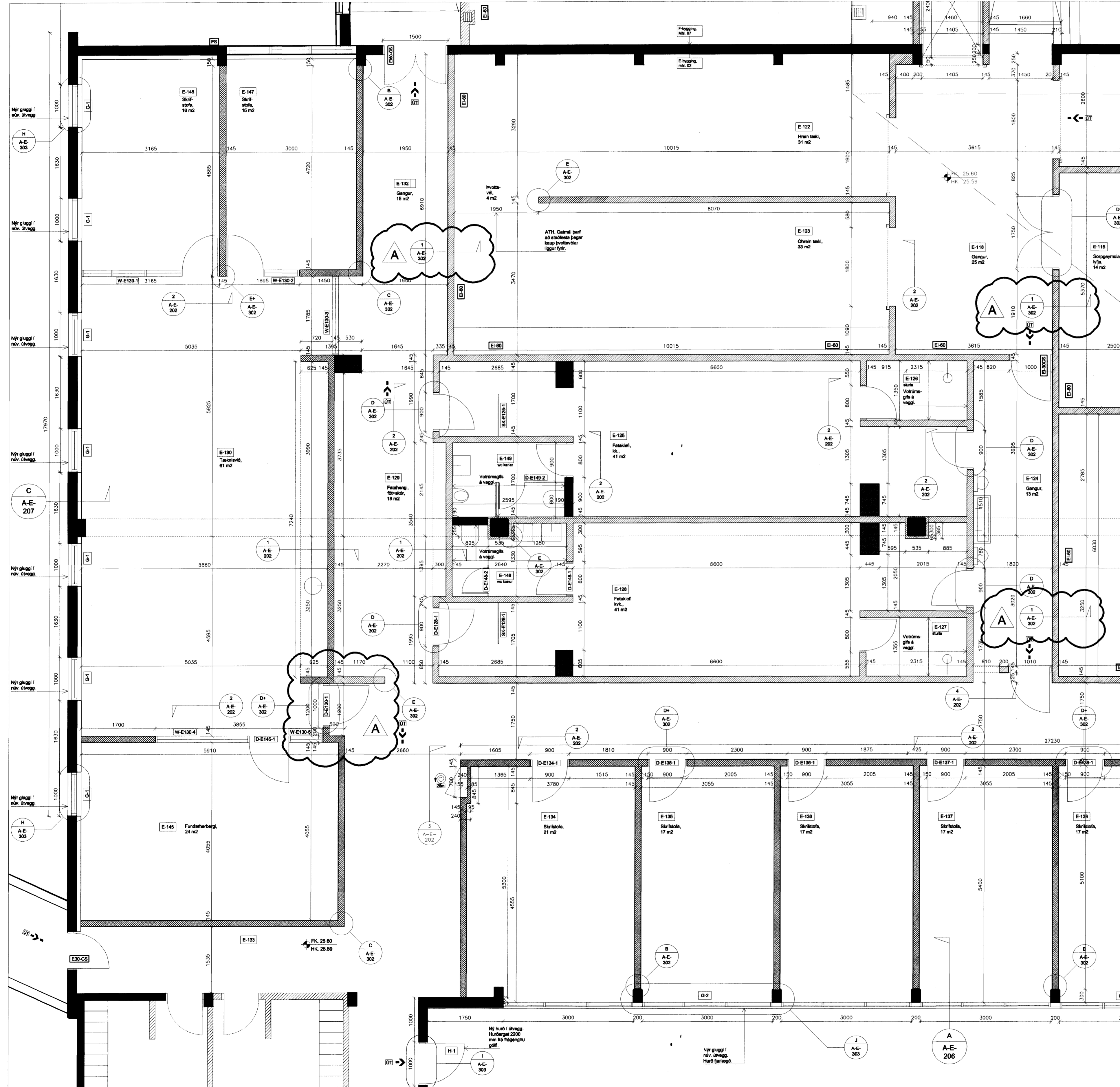
GRUNNMYND 1.HÆÐAR, 1:50
