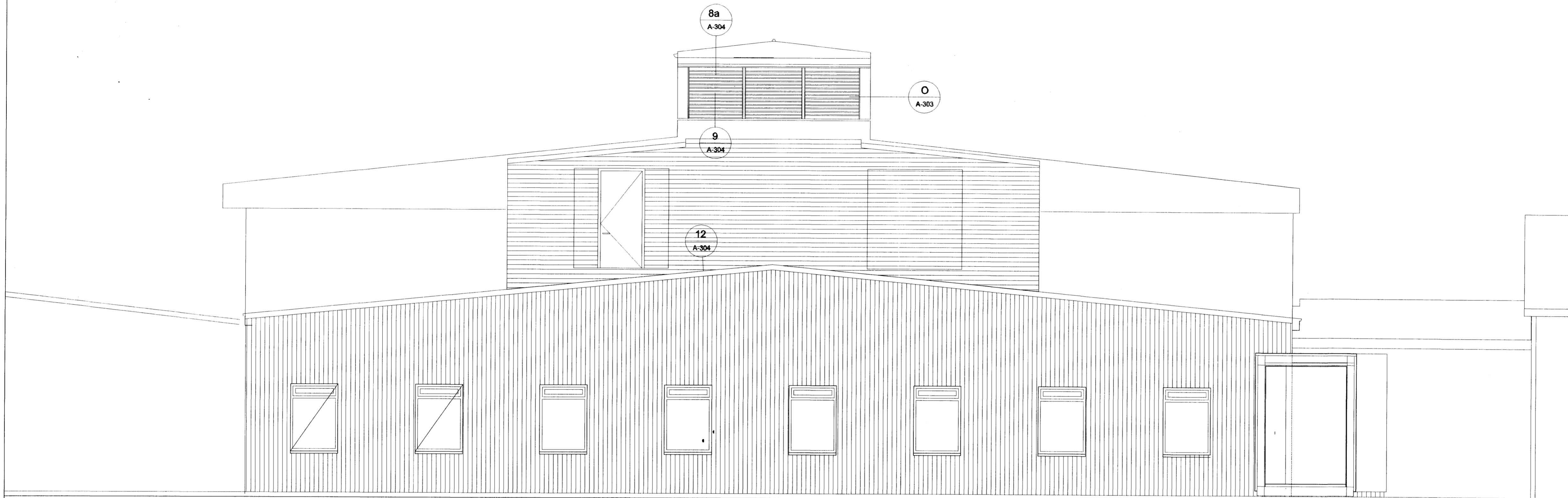
NORÐURHLIÐ 1:50
