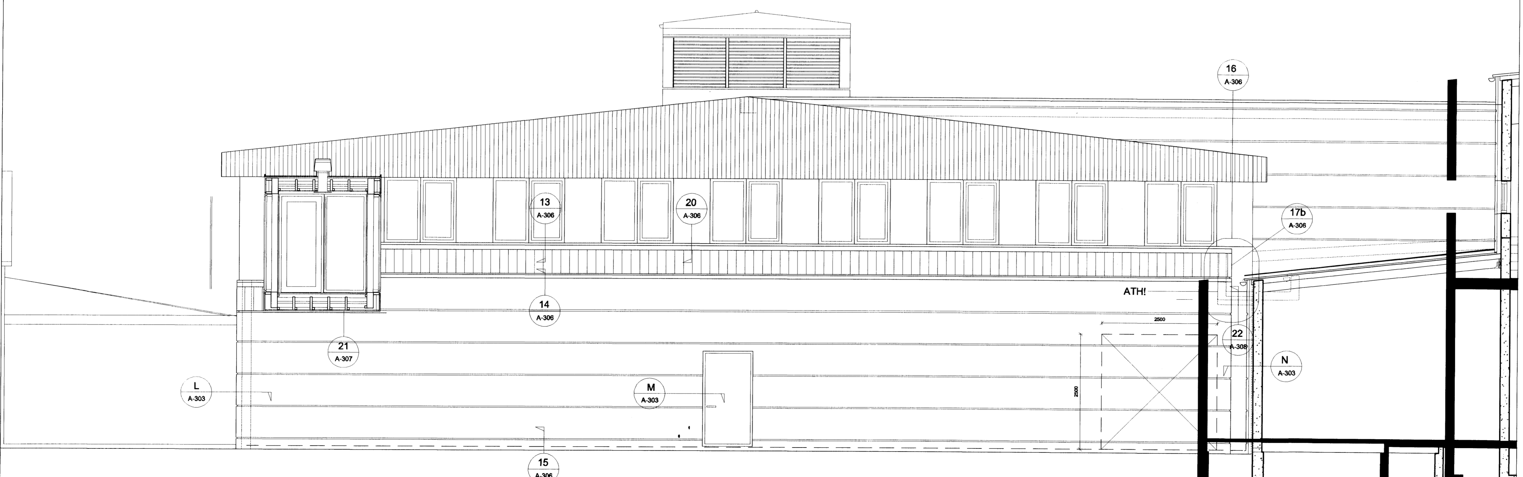
SUDURHLIÐ 1:50
