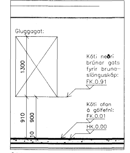
SNÍÐ 5, 1:50
