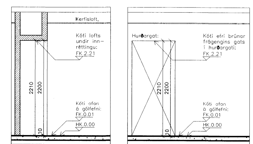
SNÍÐ 1, 1:50
