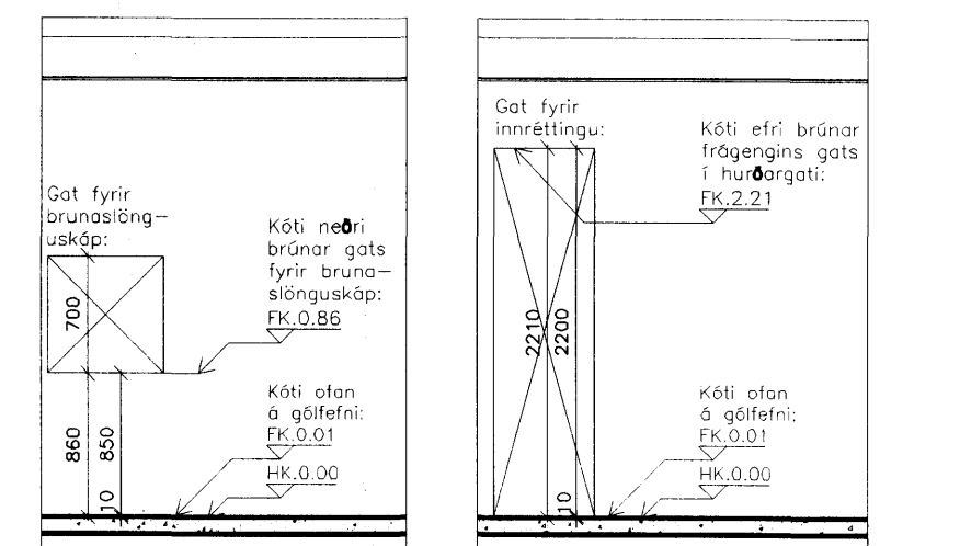
SNÍÐ 3, 1:50
