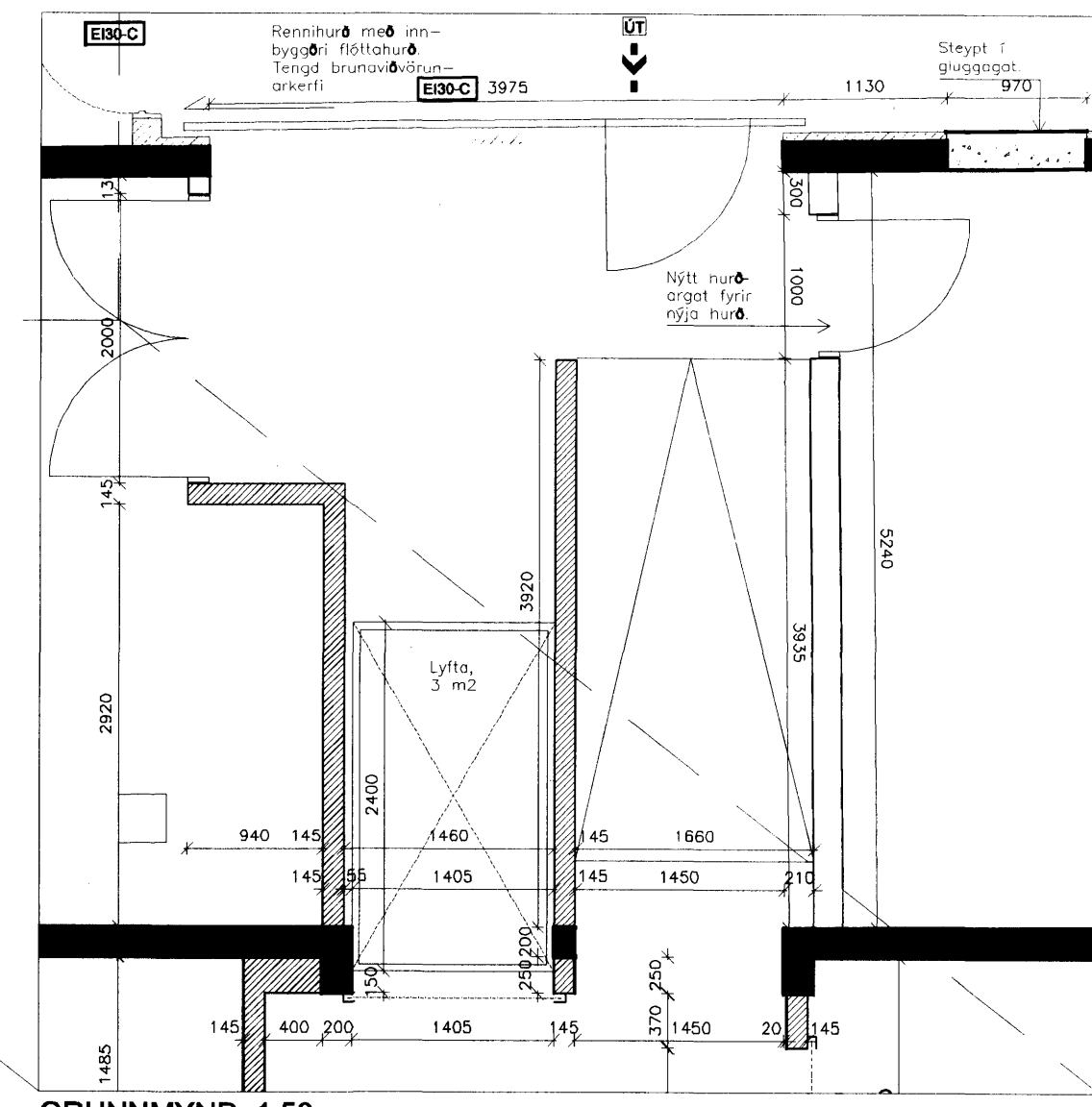
GRUNNMYND, 1:50
