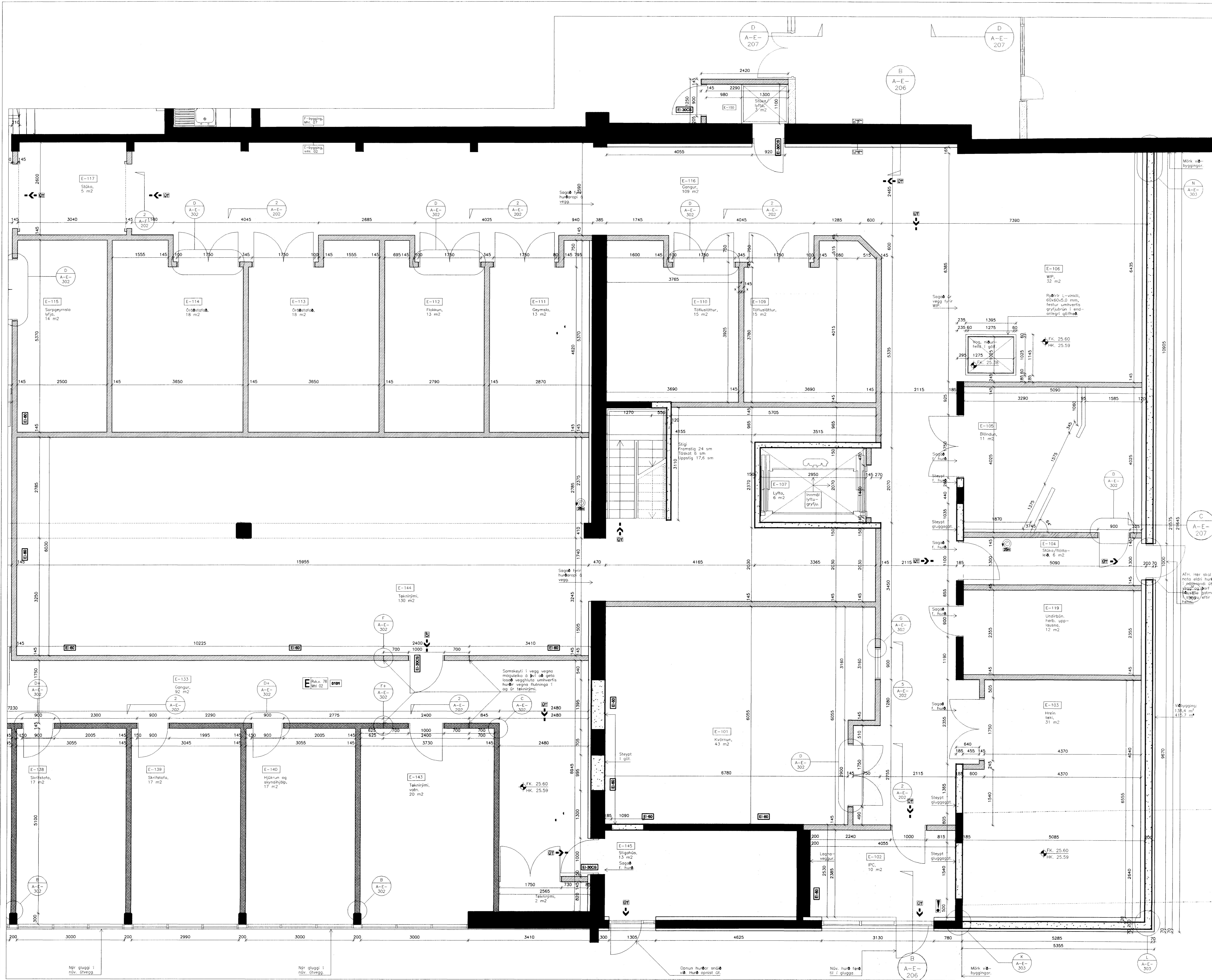
GRUNNMÝND 1.HÆÐAR, 1:50
