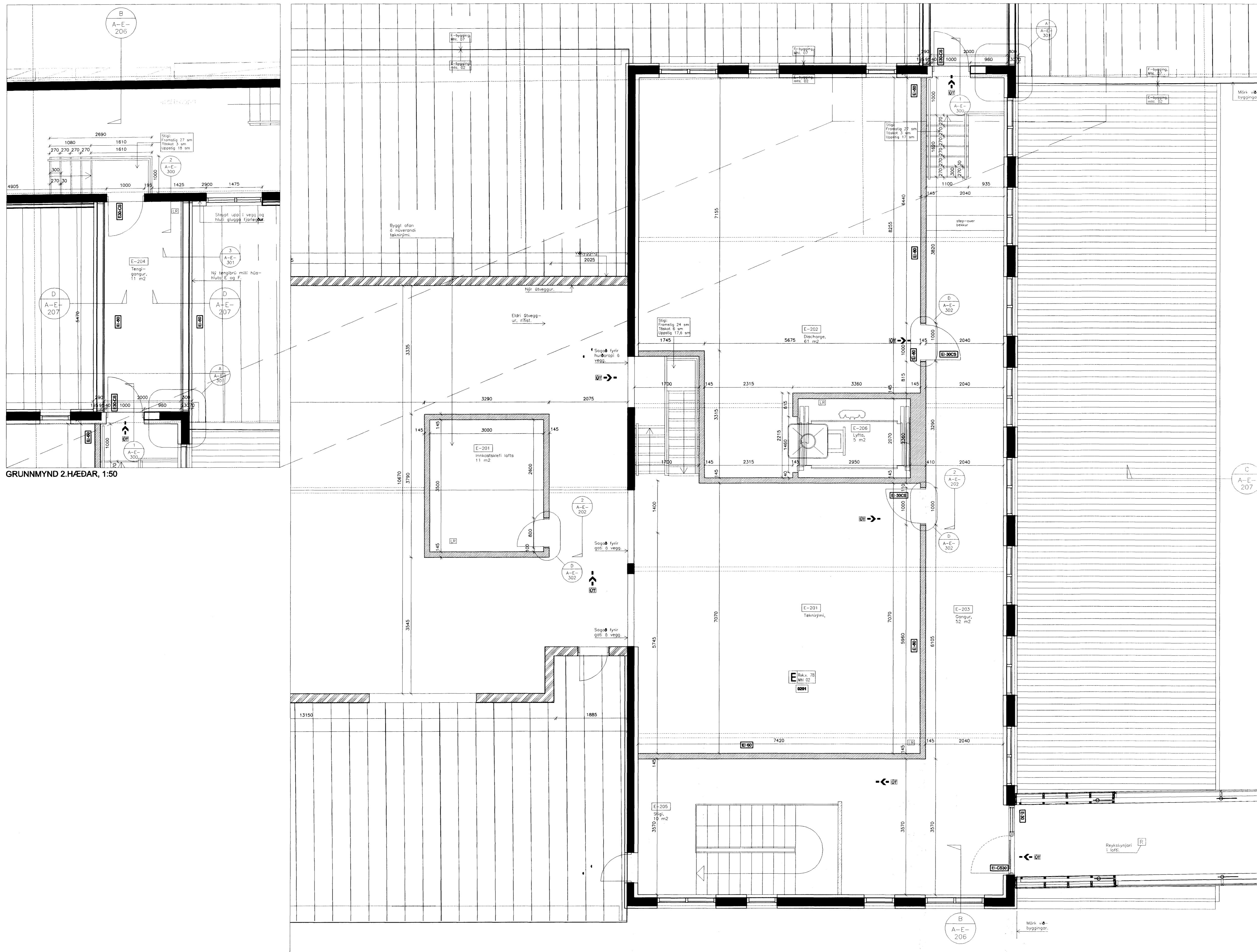
GRUNNMYND 2.HÆÐAR, 1:50
