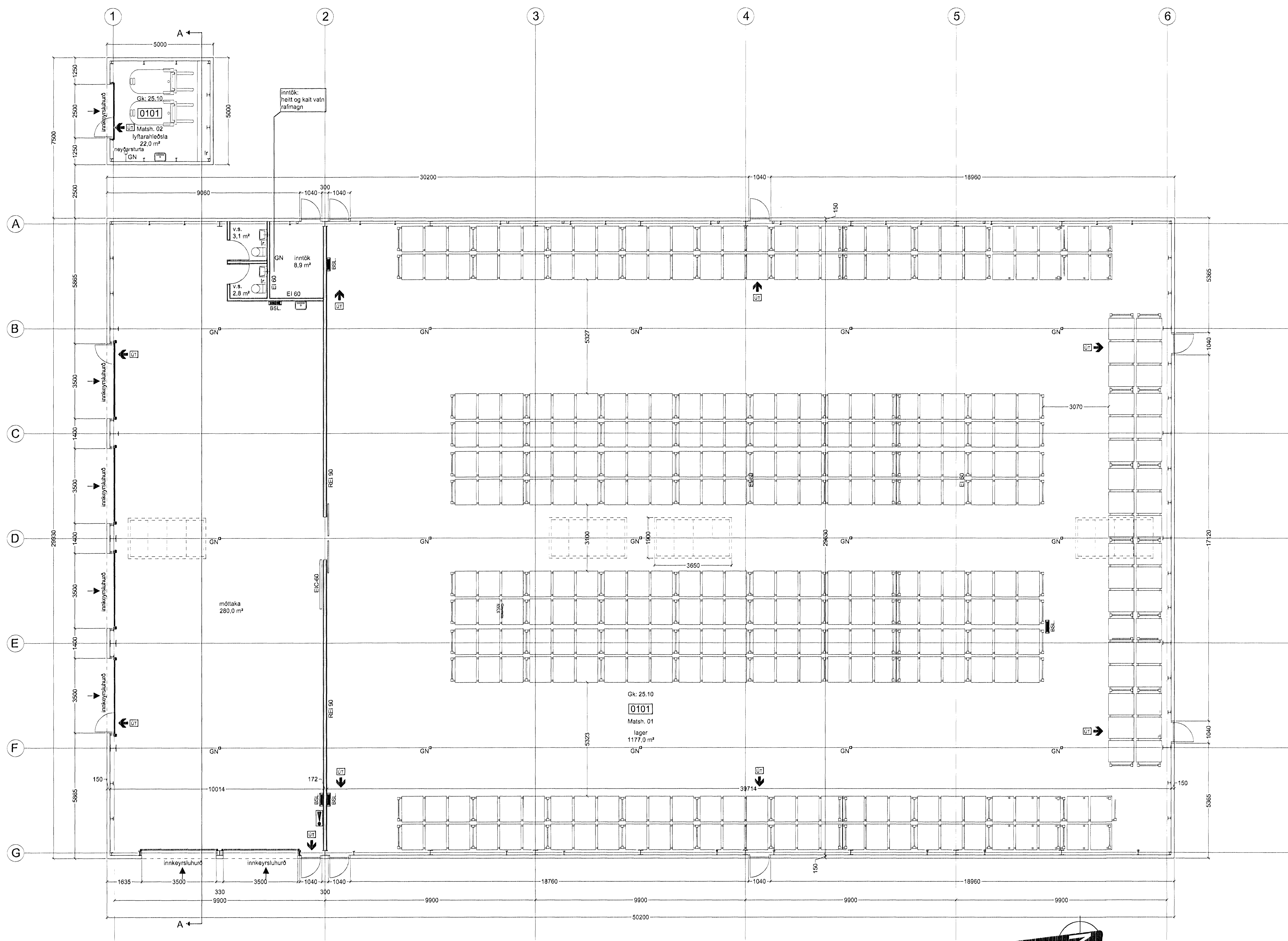
Grunnmynd 1. hæðar - 1:100
