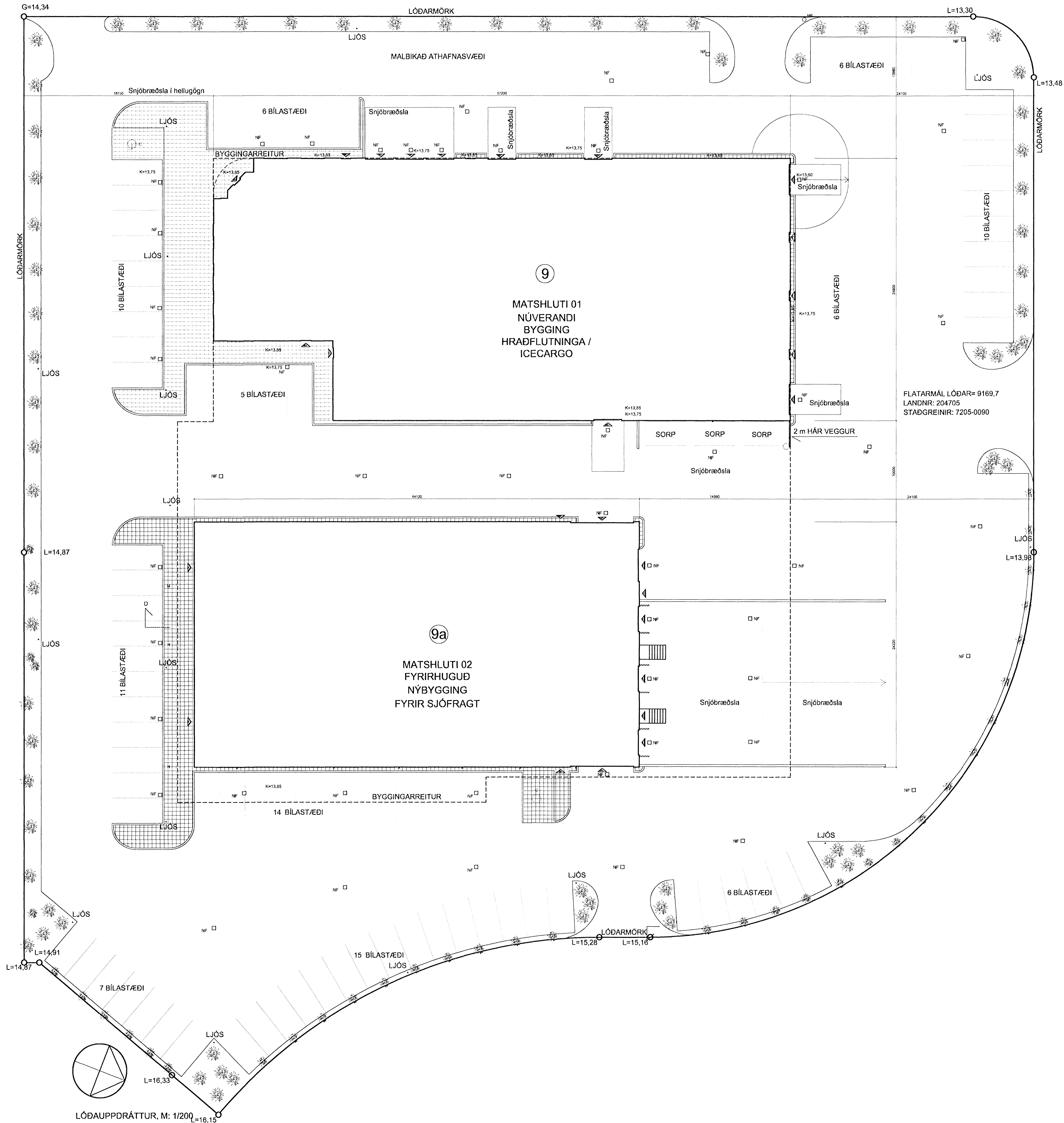
LÓÐAUPPRÁTTUR, M: 1/200
