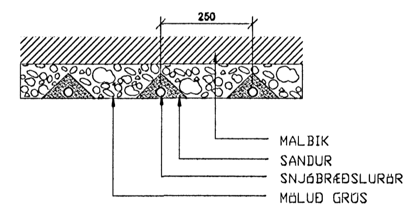
SNID Í MALBIK
