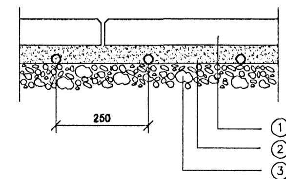
SNID Í HELLUR
