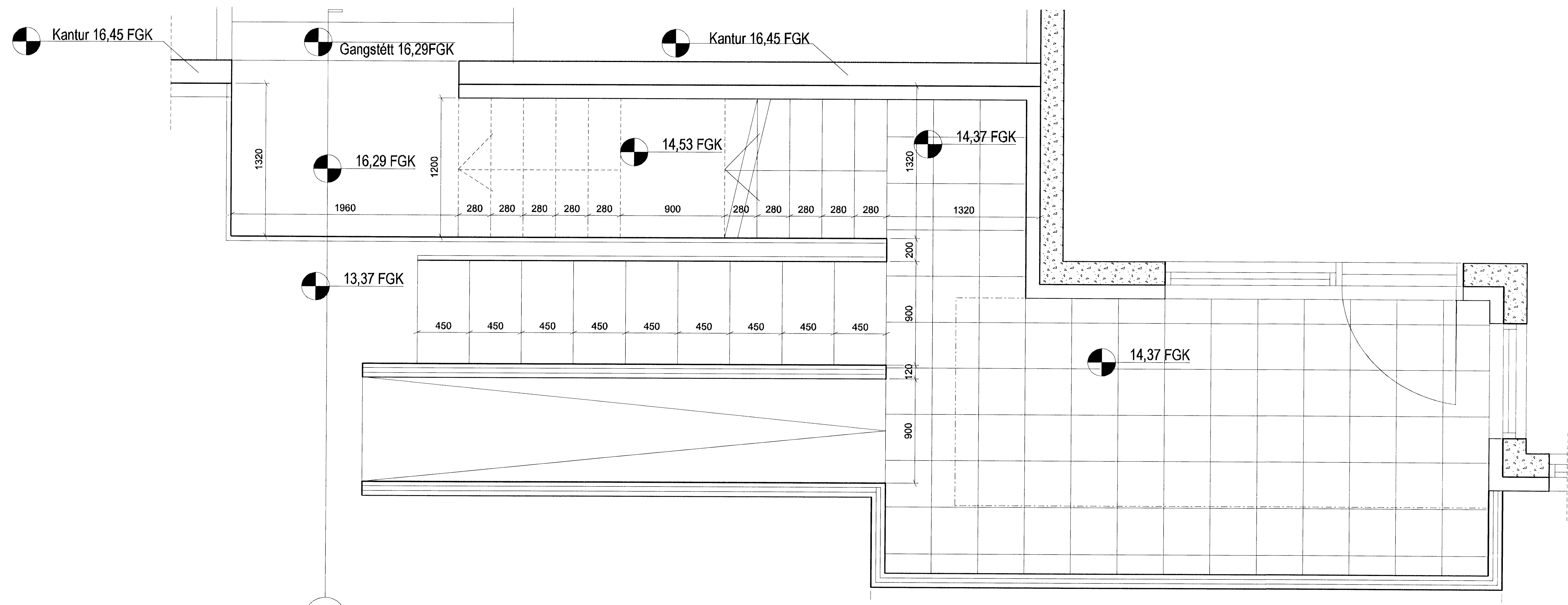
GRUNNMYND 1:20 Útiróppur
