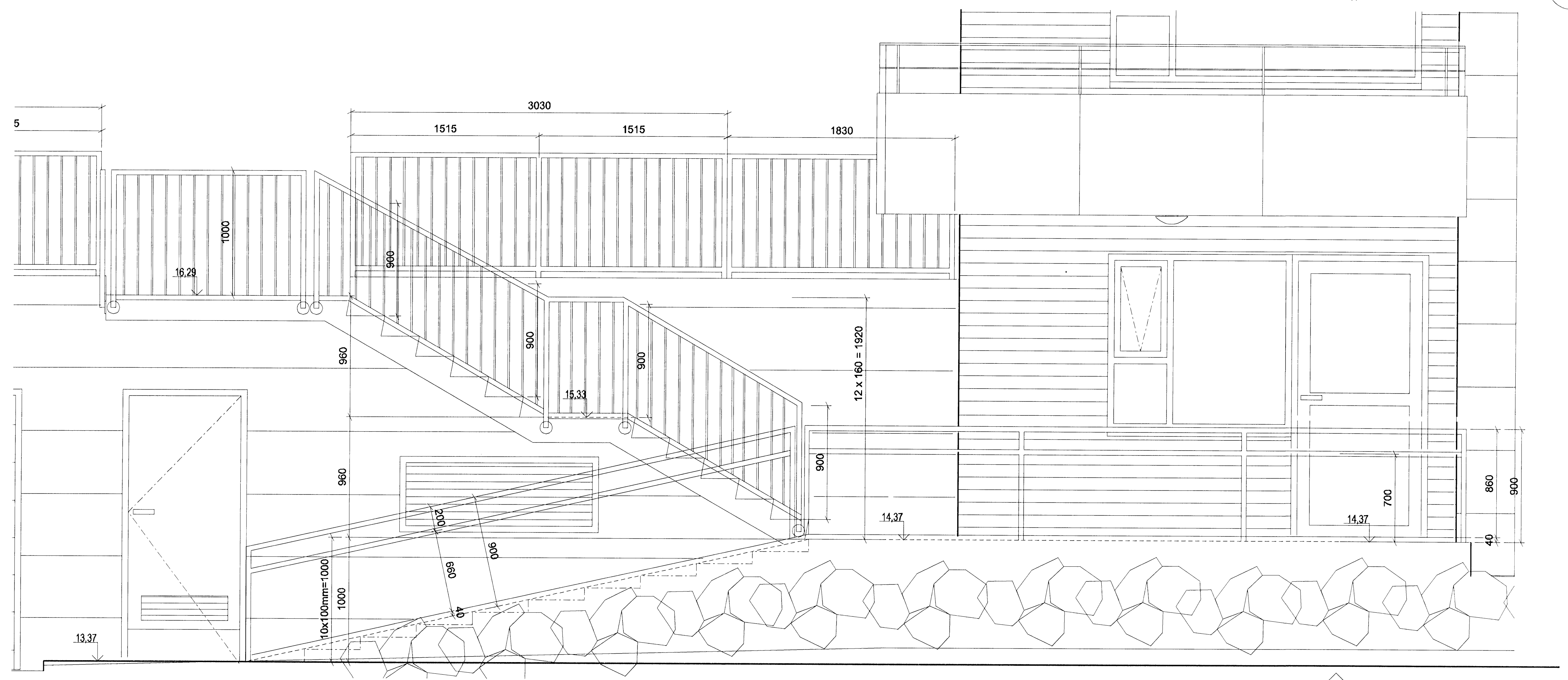
ÚTLIT 1:20 Útiróppur
