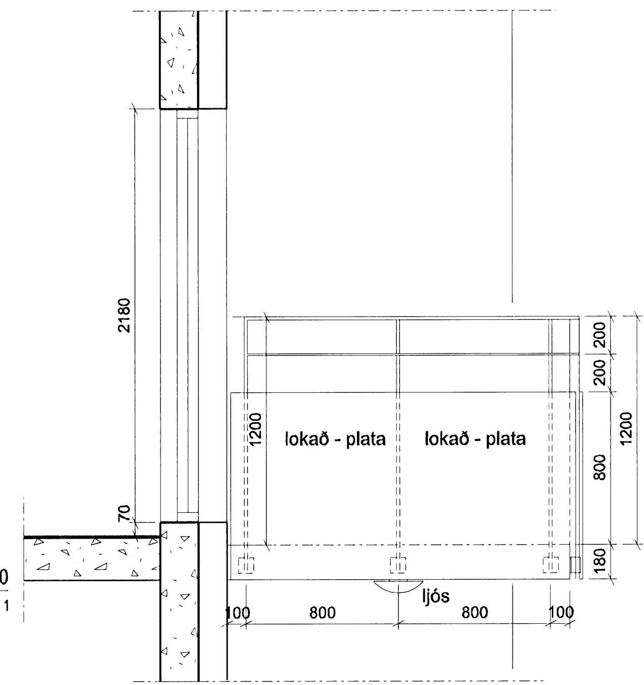
SNEIÐING 1:20 útlit af svölum grm. nr. 1
