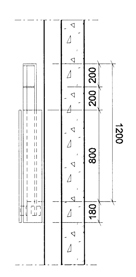
SNEIÐING 1:20 útlit af svölum grm. nr. 2
