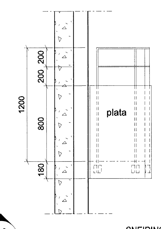
SNEIÐING 1:20 útlit af svölum grm. nr. 2
