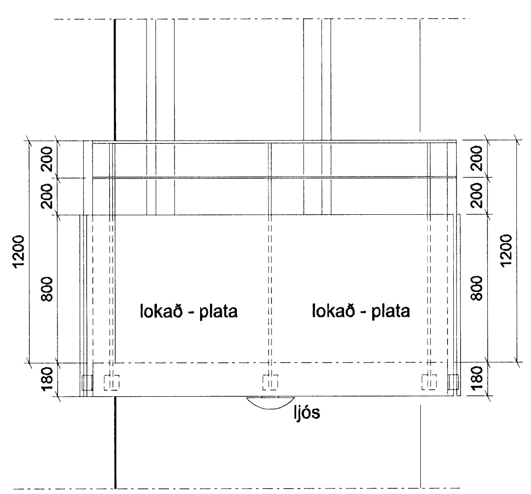
SNEIÐING 1:20 útlit af svölum grm. nr. 2
