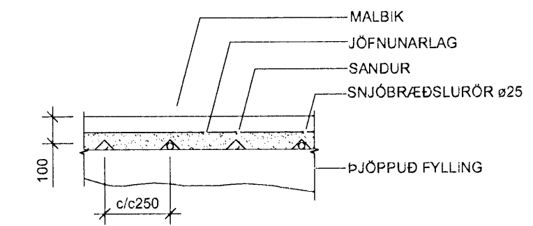
SM1 SÉRMYND 1:20
