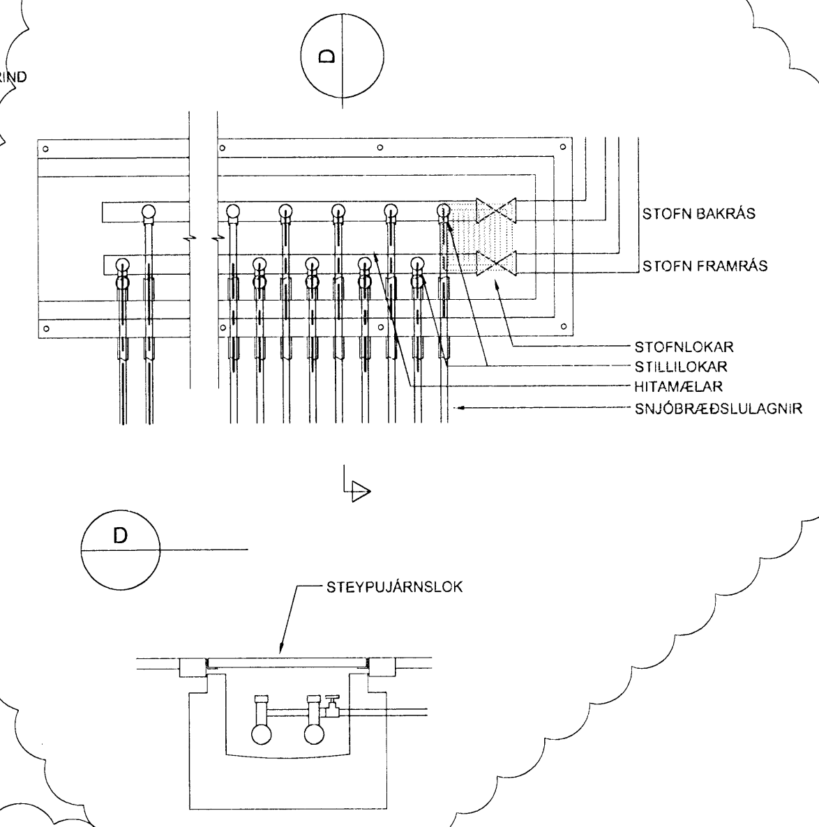
SM1 SÉRMYND 1:20
