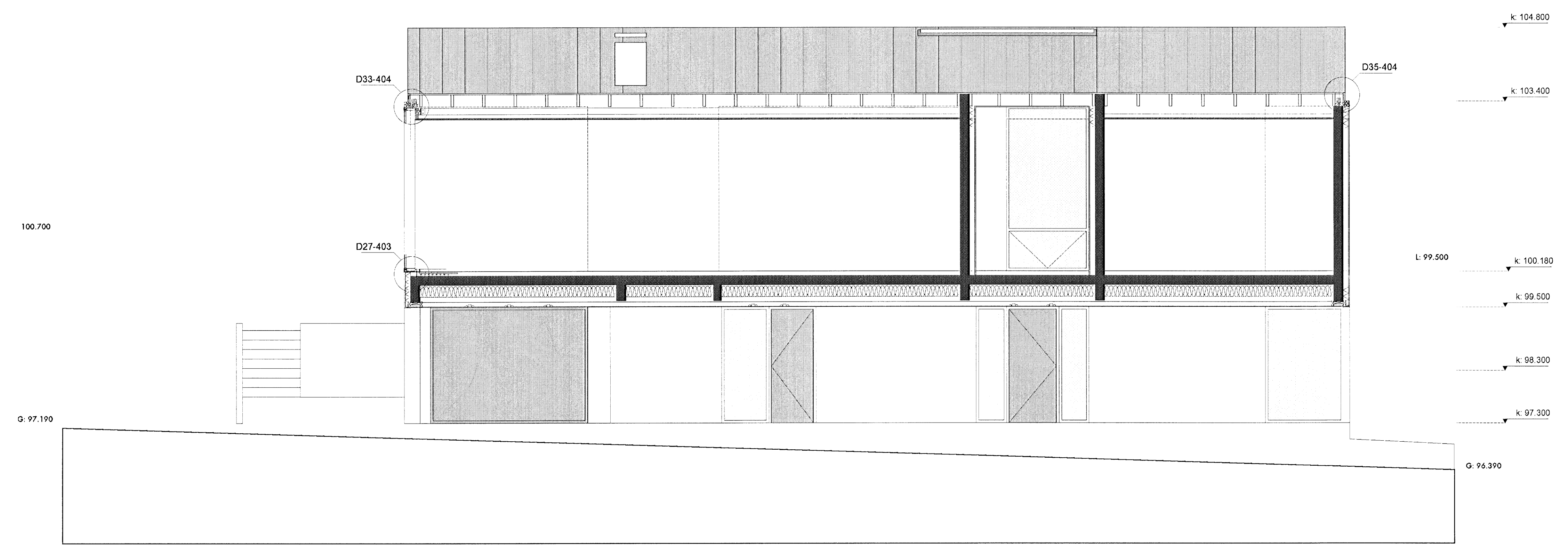
skurður DD 1:50
