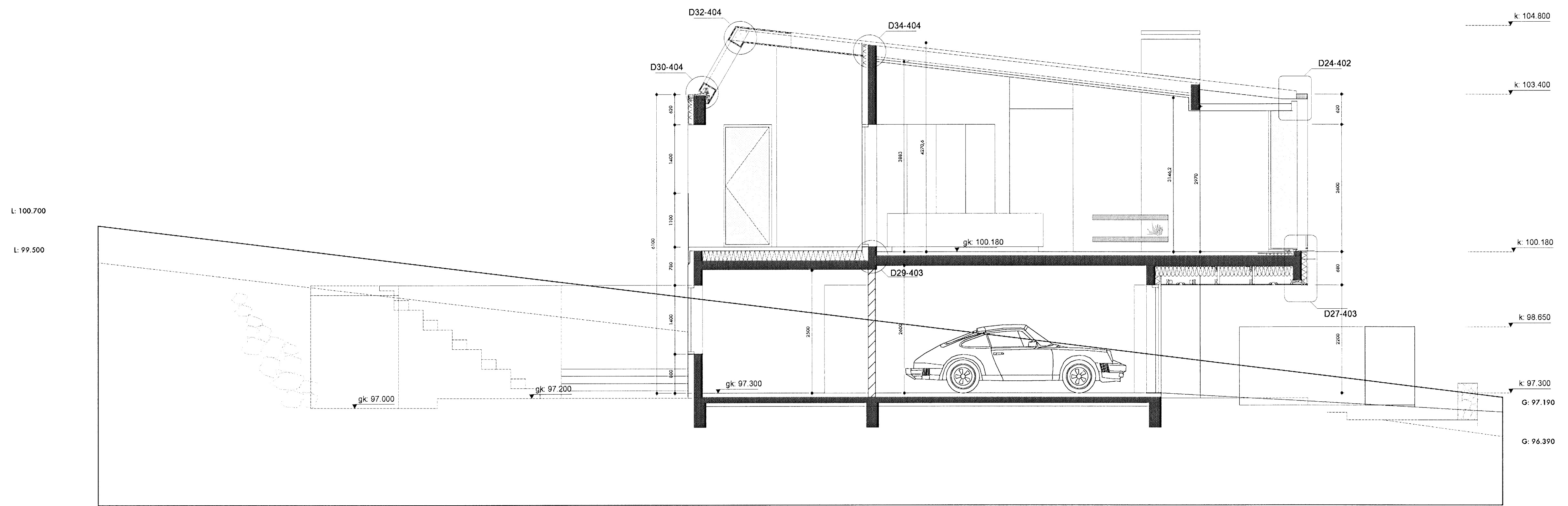
skurður CC 1:50
