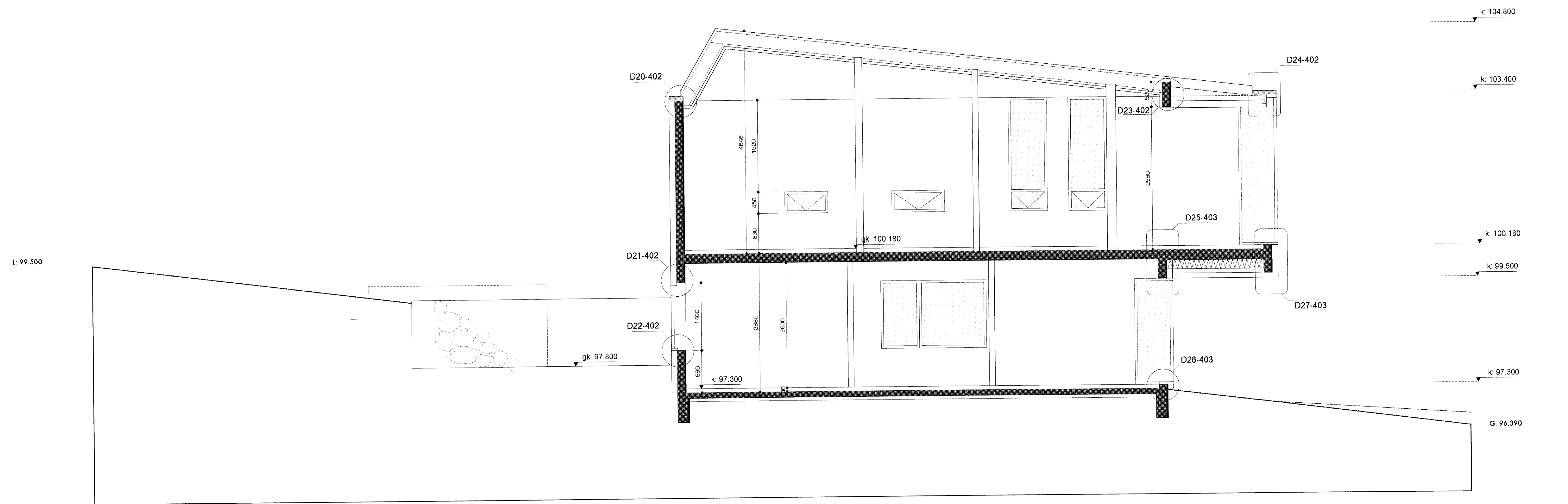
skurður AA 1:50
