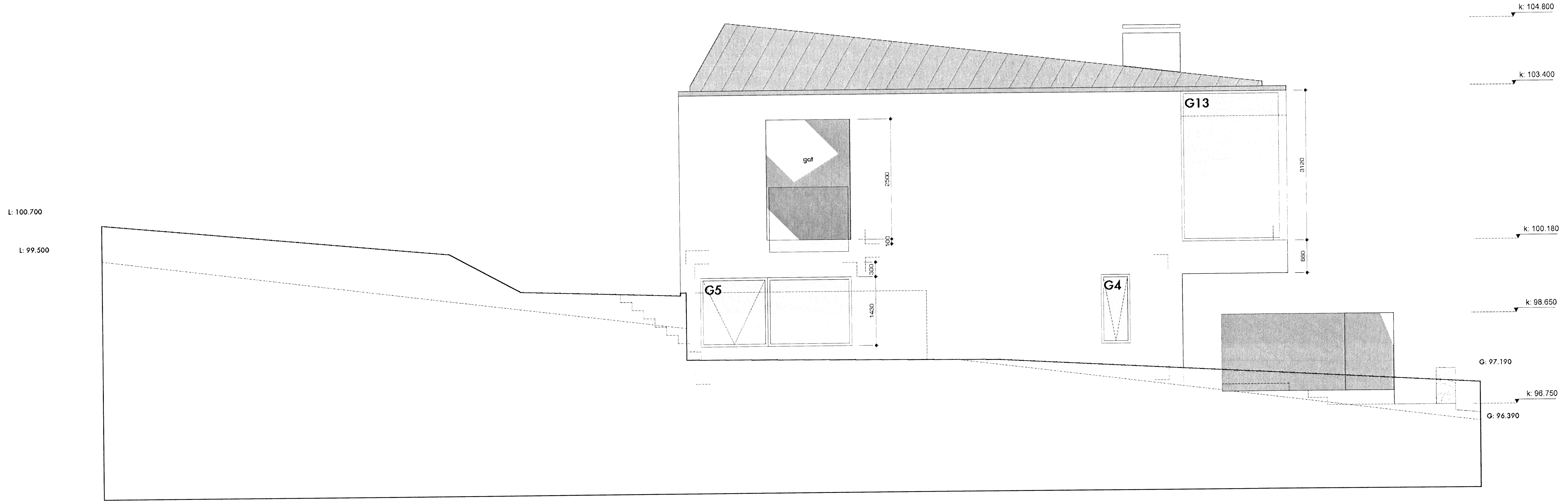
útlit suður 1:50
