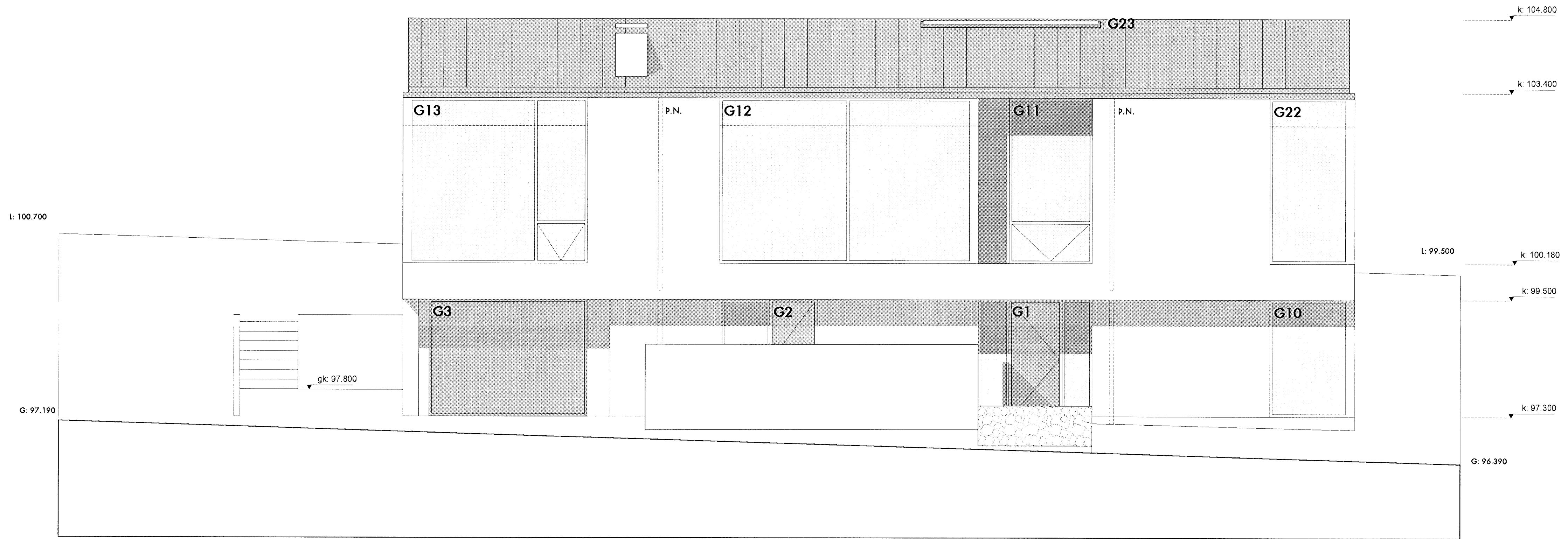
Útlit austur 1:50
