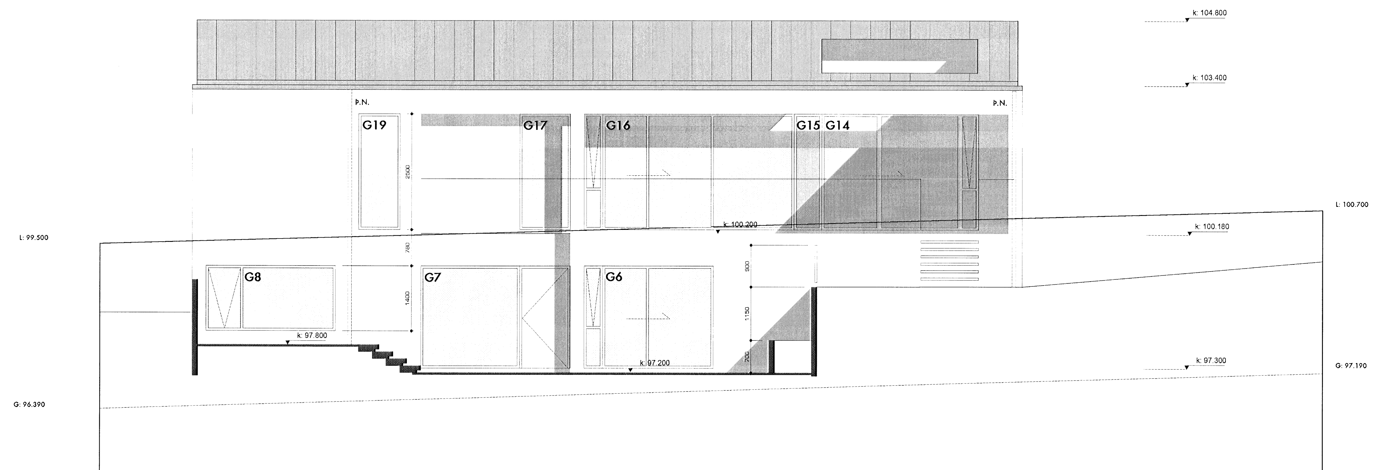
Útlit vestur 1:100
