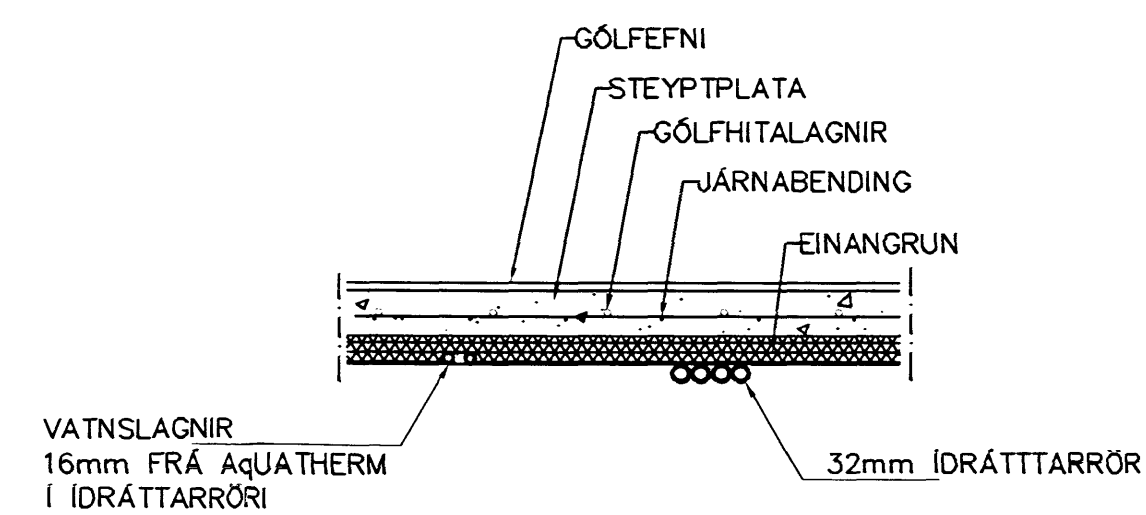
LAGNIR, SNIÐ, 1:20
