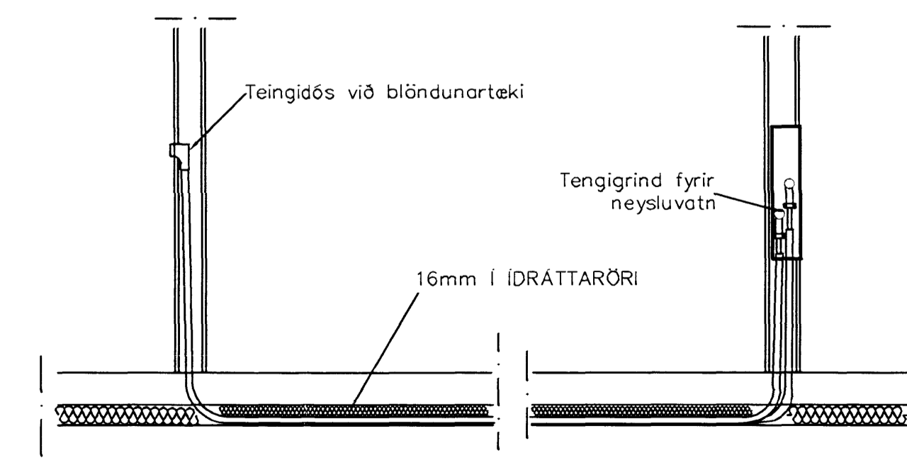
TENING NEYSLUVATNSLAGNA 1:20
