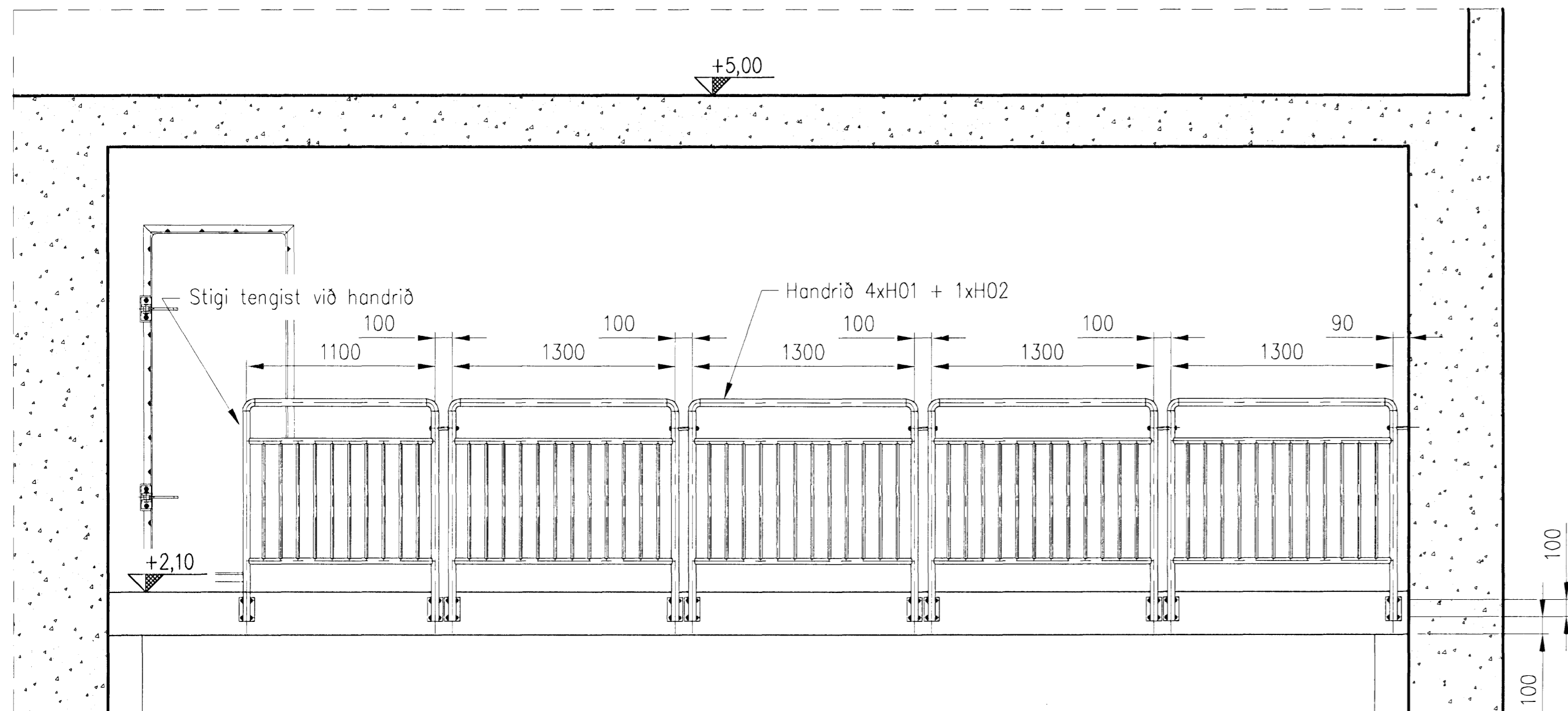
HANDRIÐ H01 Á SVÖLUM Í SKOLPRÝMI
