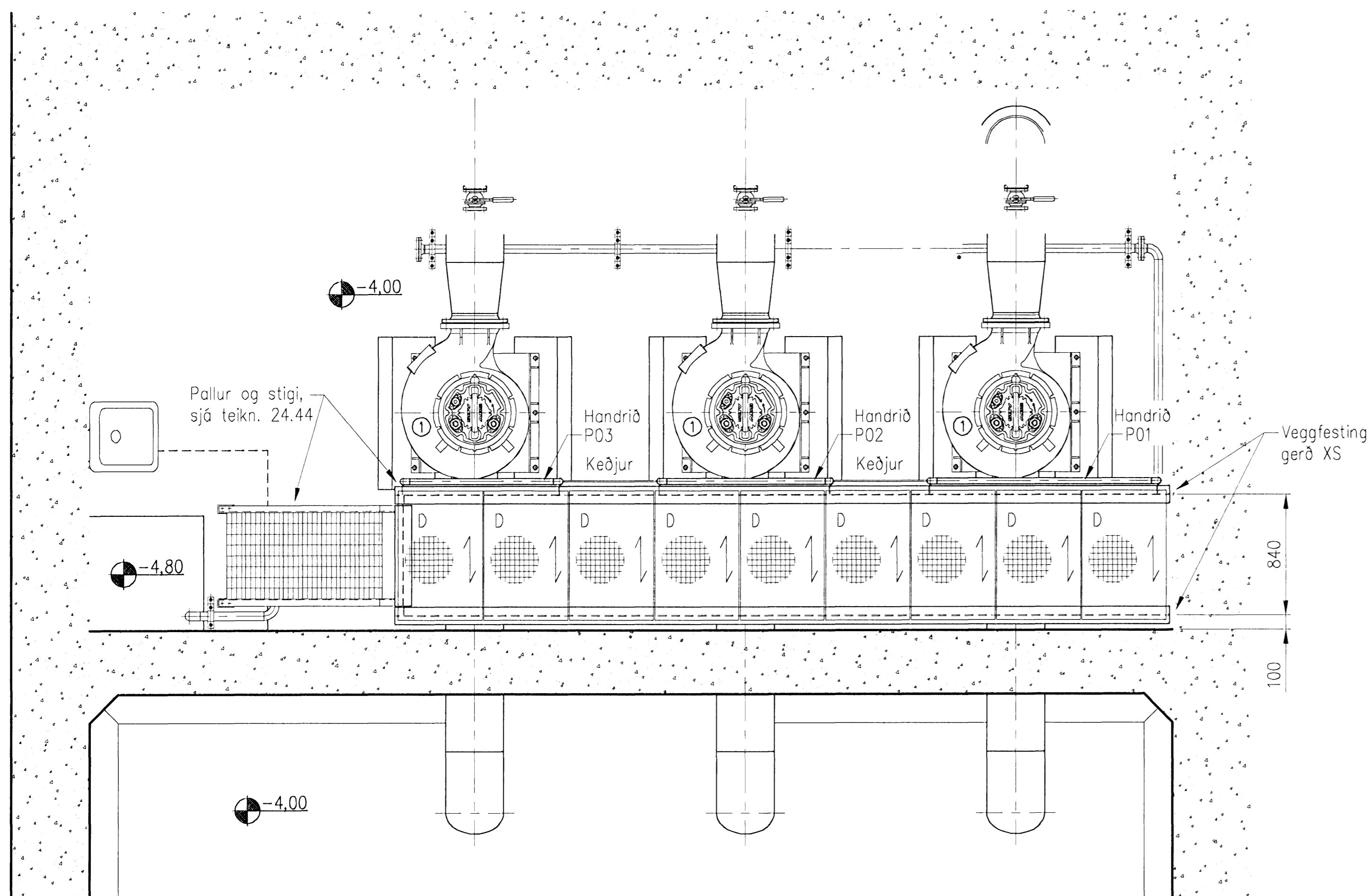
LÁRÉTT SNIÐ Í DÆLURÝMI
