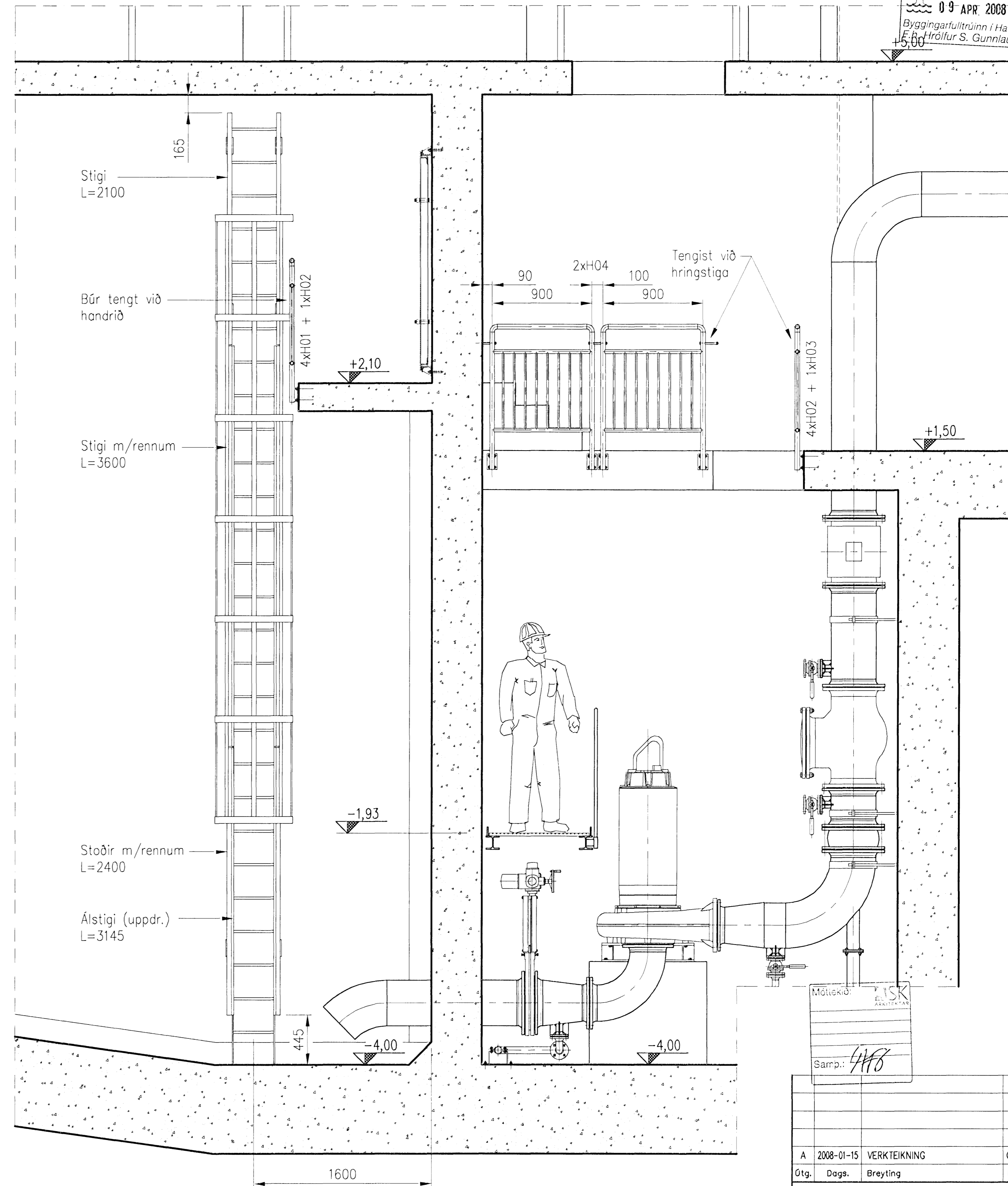
LÓDRÉTT SNIÐ Í SKÓLP- OG DÆLURÝMI
