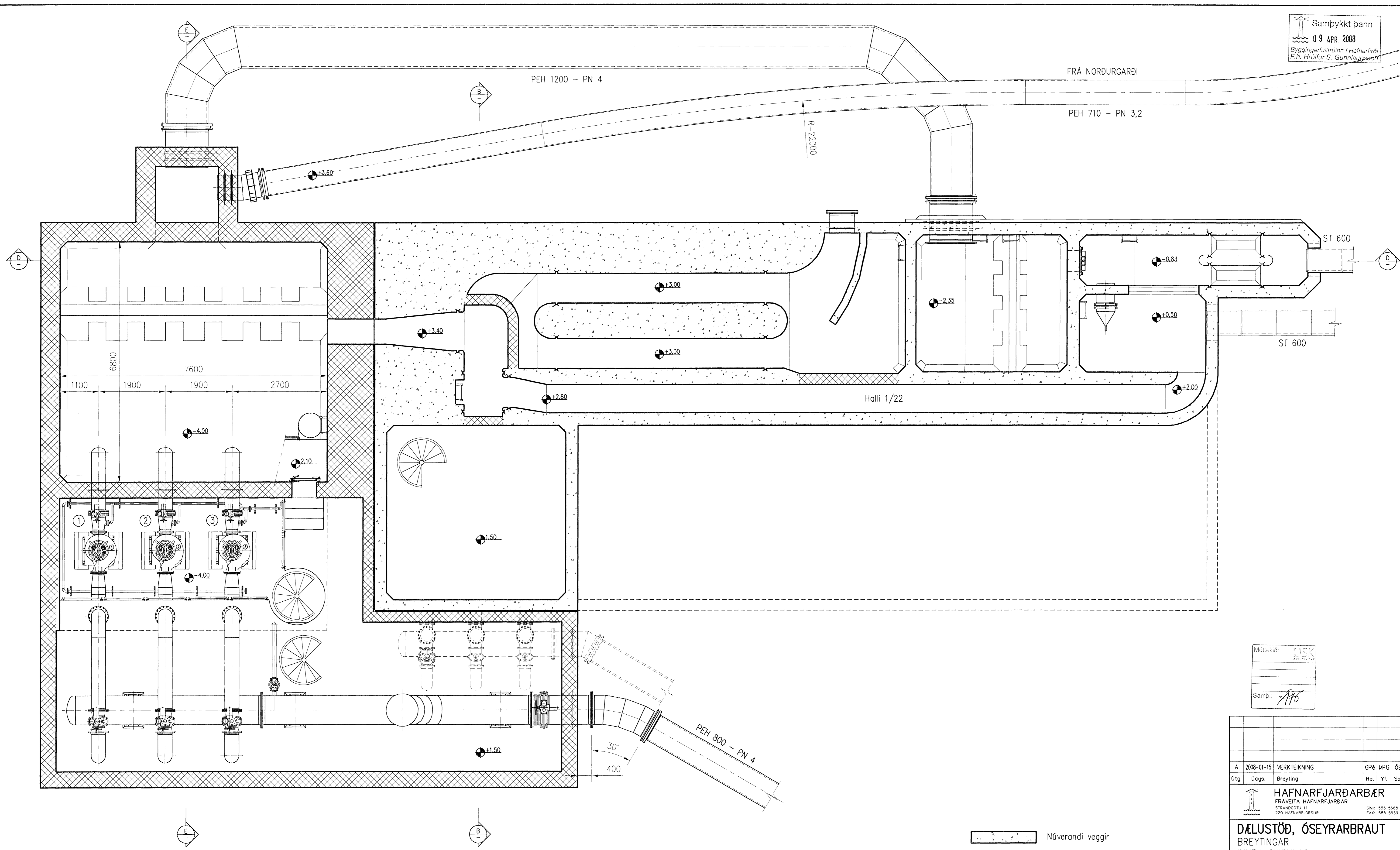
GRUNNMYND NEDRI HÆÐAR
