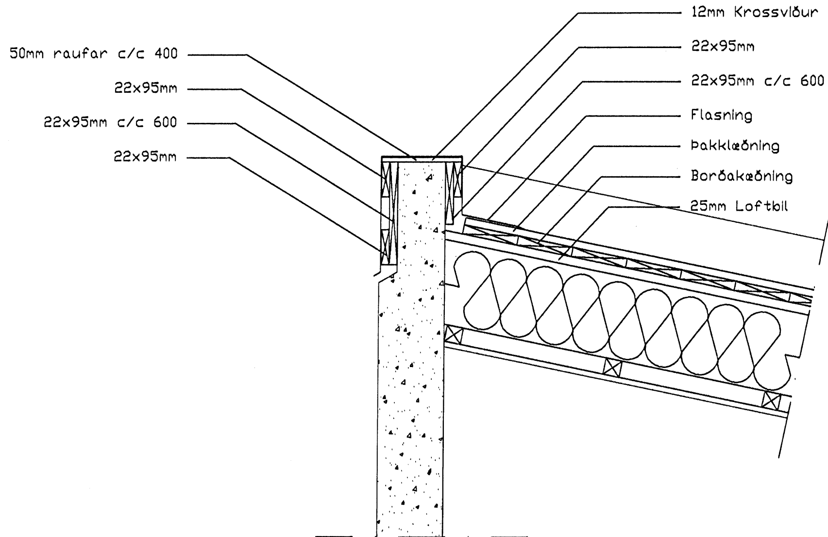
SNID Í ÞAK MKV. 1:10
