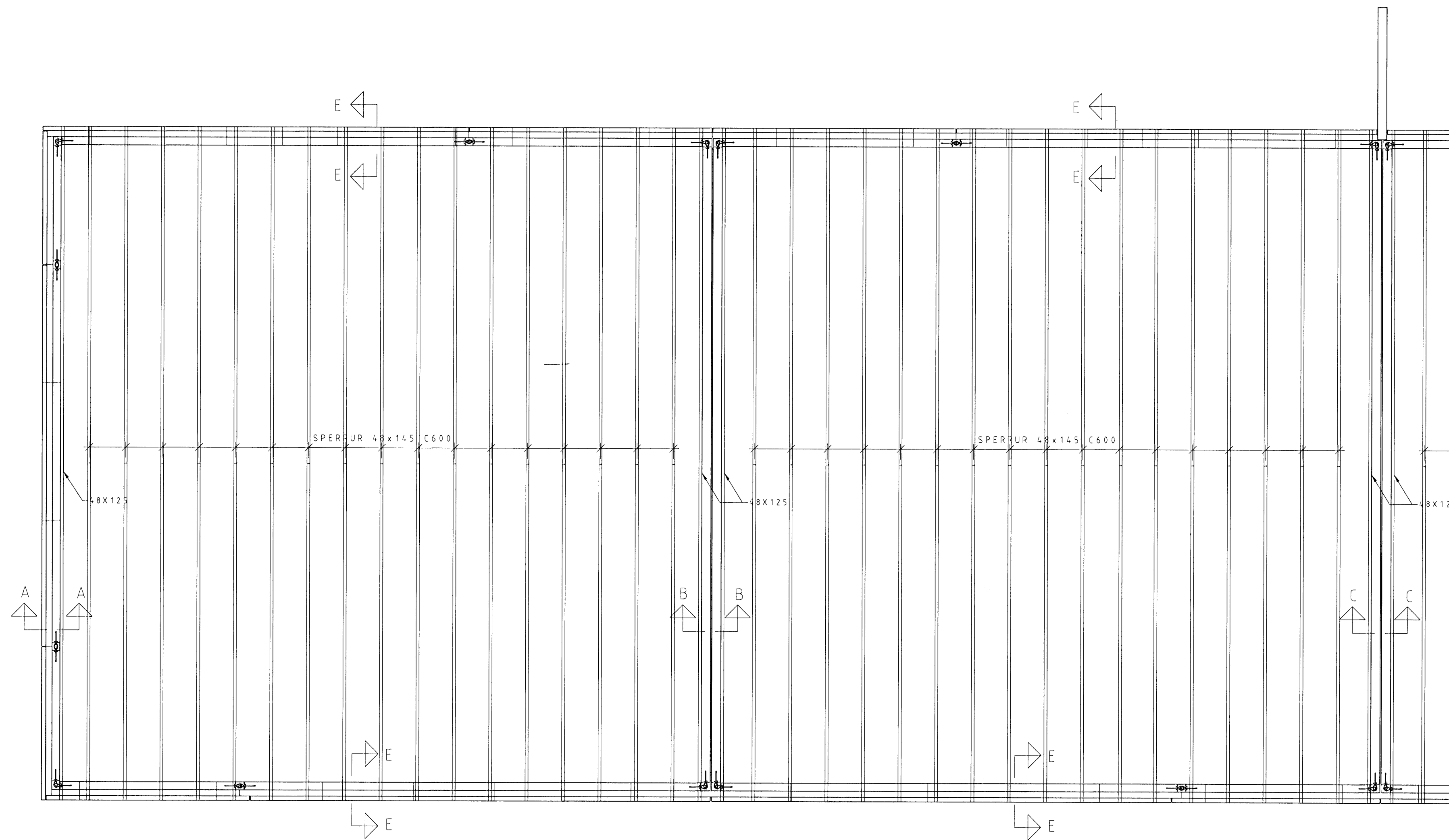
SPERRUPLAN 1:50
