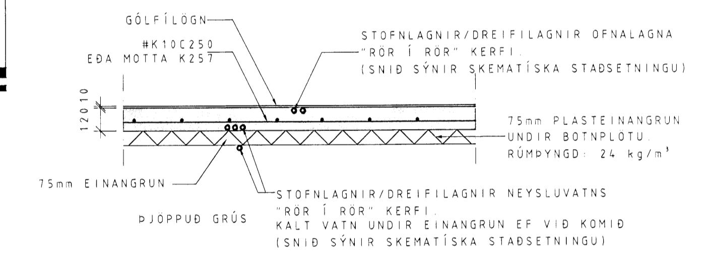
ALMENNT SNID Í BOTNPLÖTU 1:20
