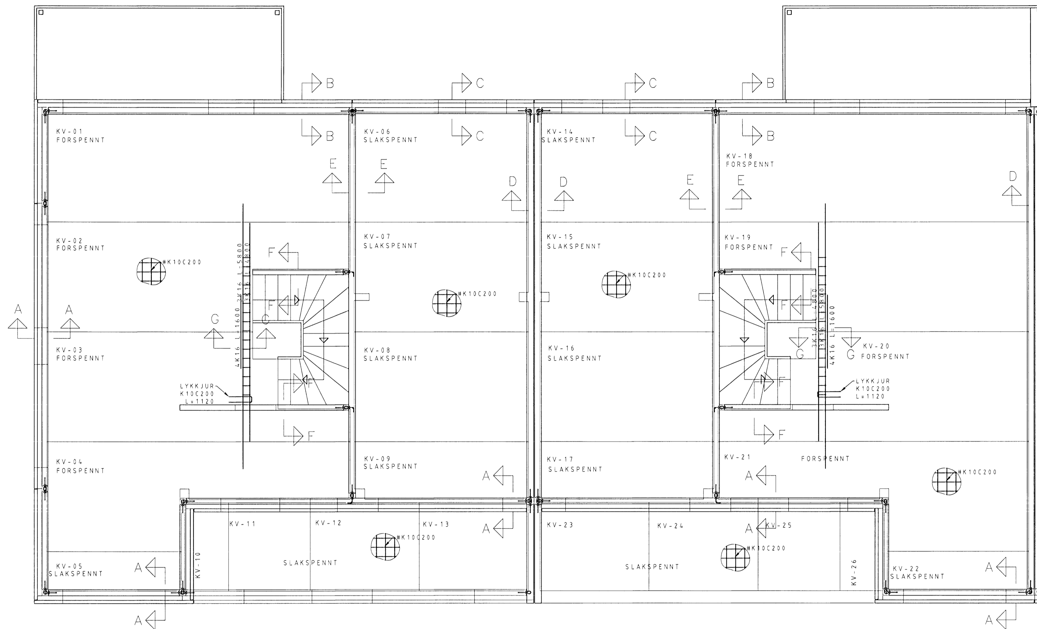
GRUNNMYND VEGGJA 1.HÆÐ 1:50
