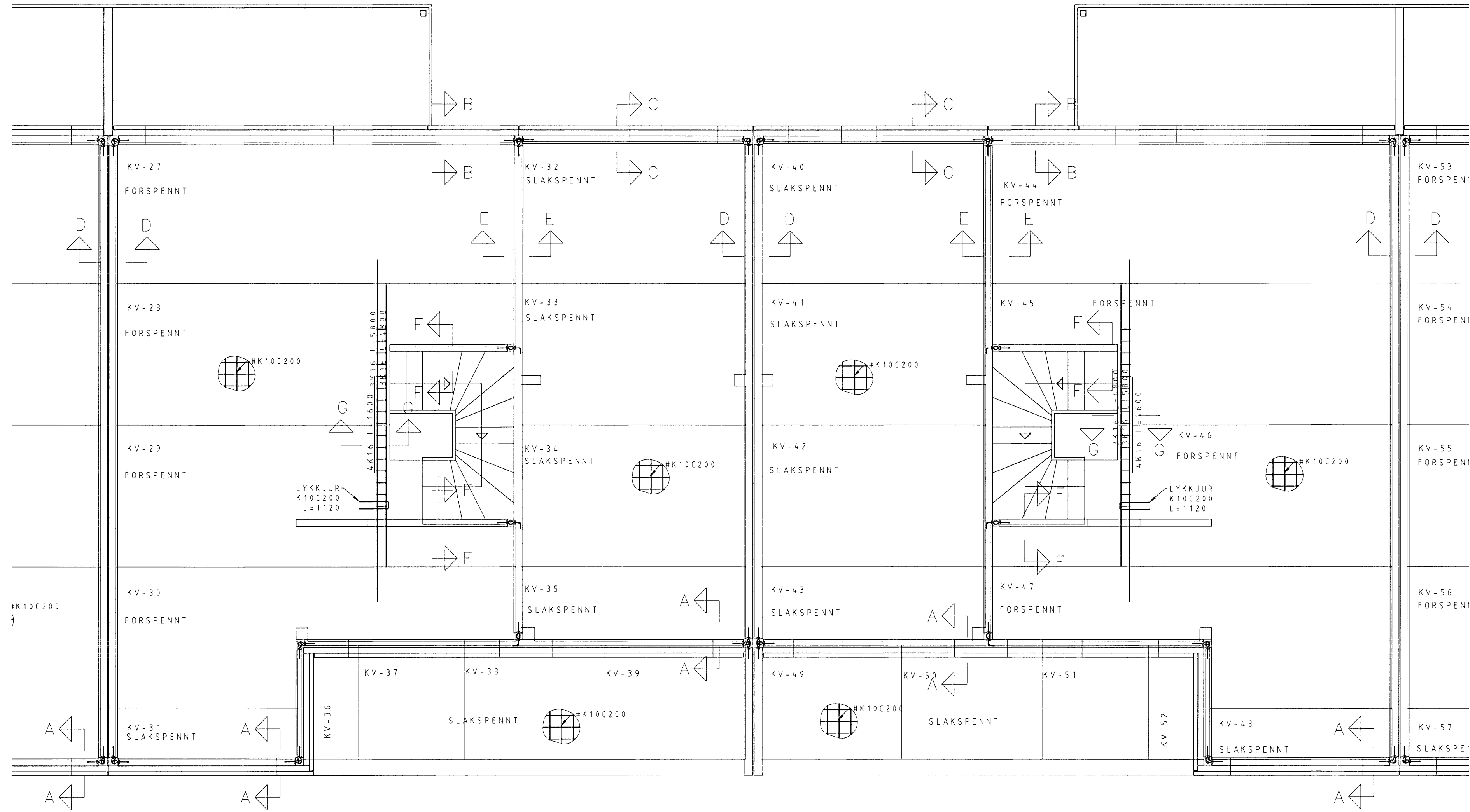
GRUNNMYND VEGGJA 1.HÆÐ 1:50
