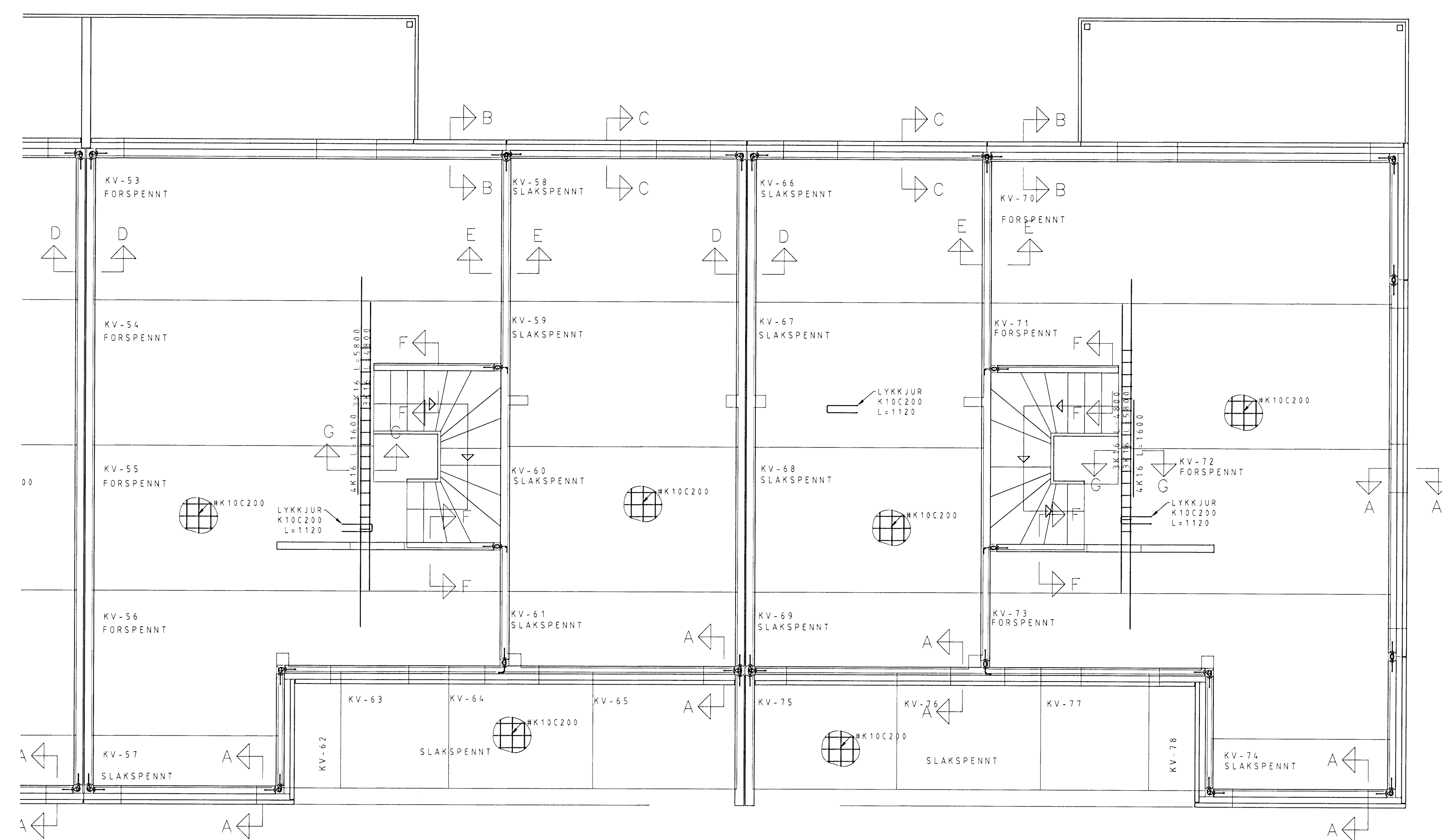
GRUNNMYND VEGGJA 1. HÆÐ 1:50
