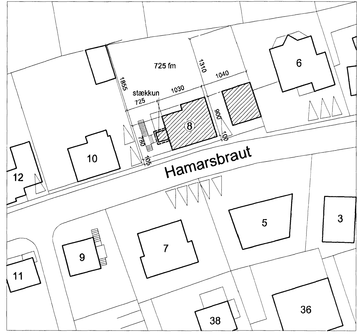
Afstöðumynd - 1:500
