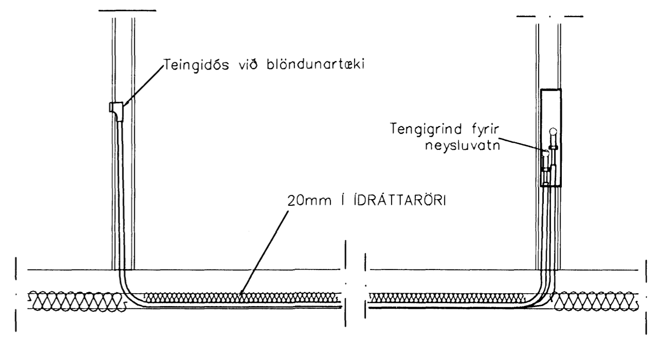
TENING NEYSLUVATNSLAGNA 1:20
