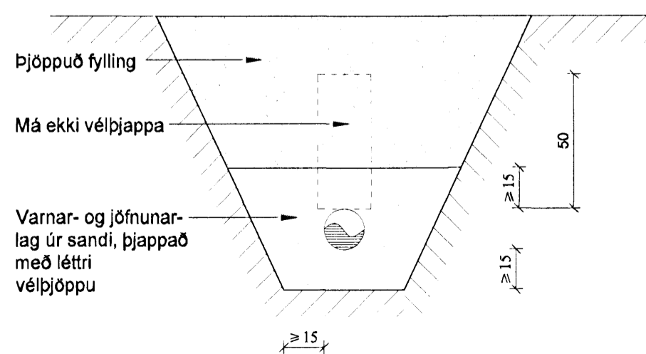
Frárennslislagnir í jörðu og grunni. 1:20
