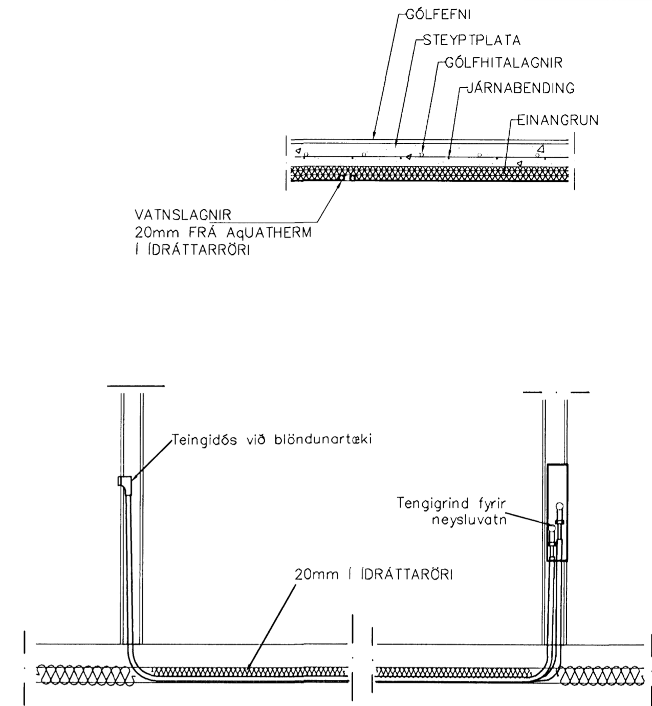
TENING NEYSLUVATNSLAGNA 1:20
