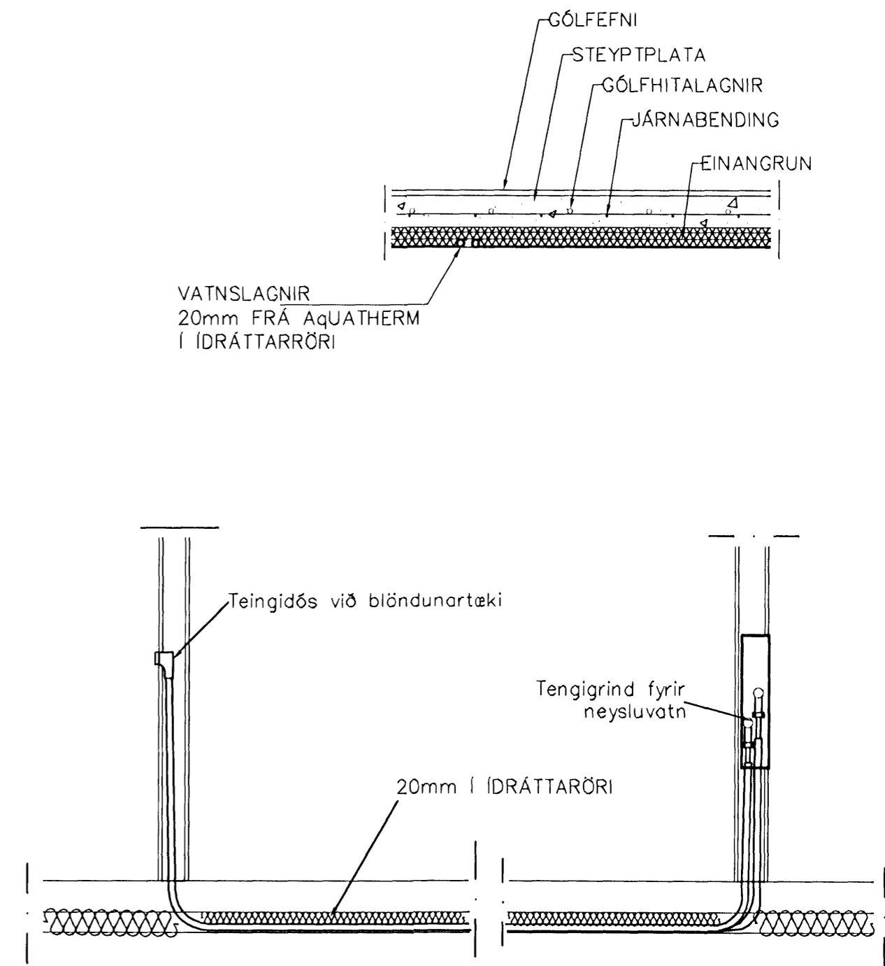
TENING NEYSLUVATNSLAGNA 1:20
