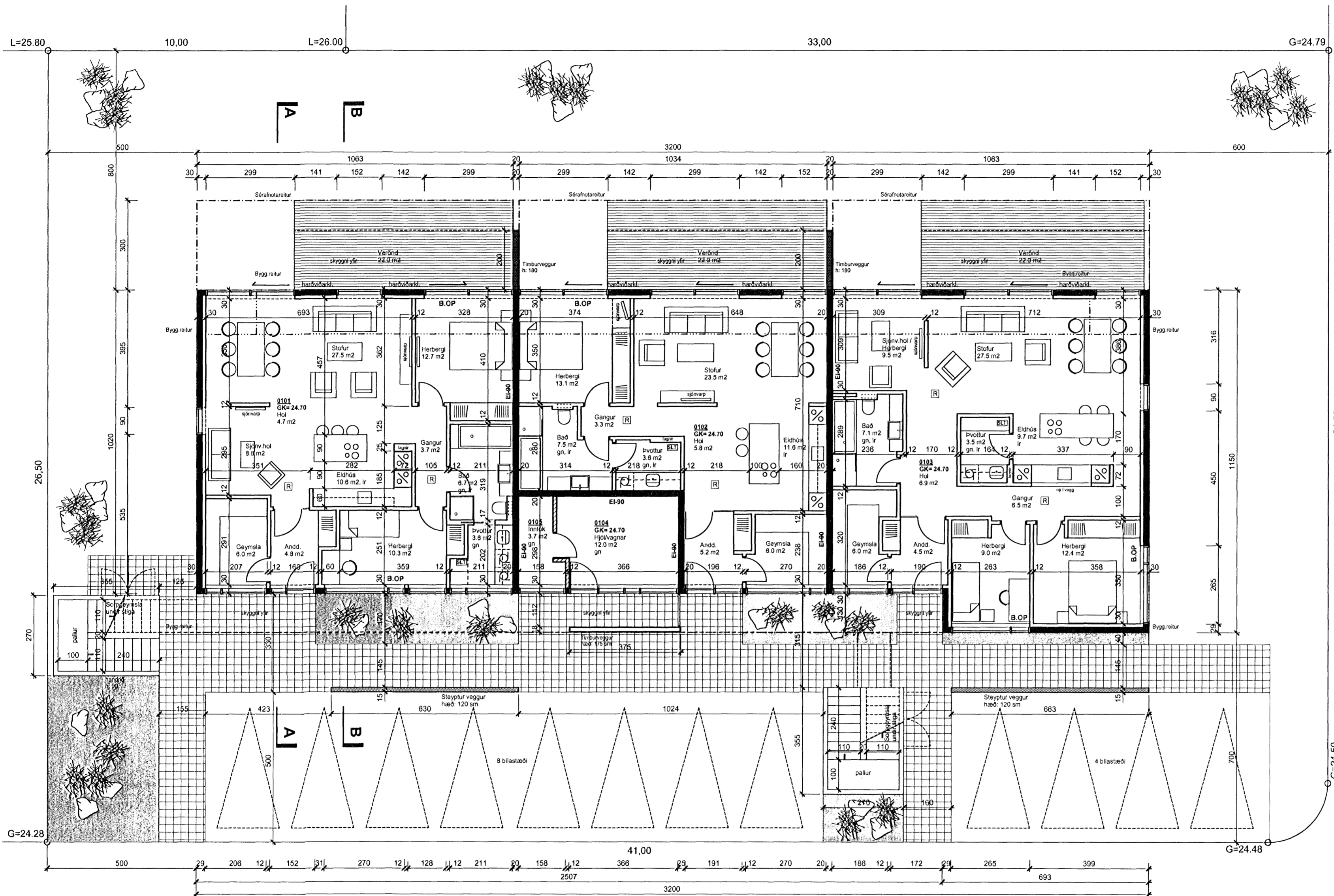
GRUNNMYND 1.HÆÐAR
