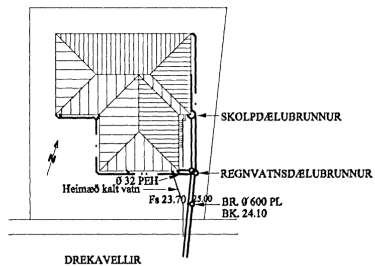
AFSTÖÐUMYND 1:500
