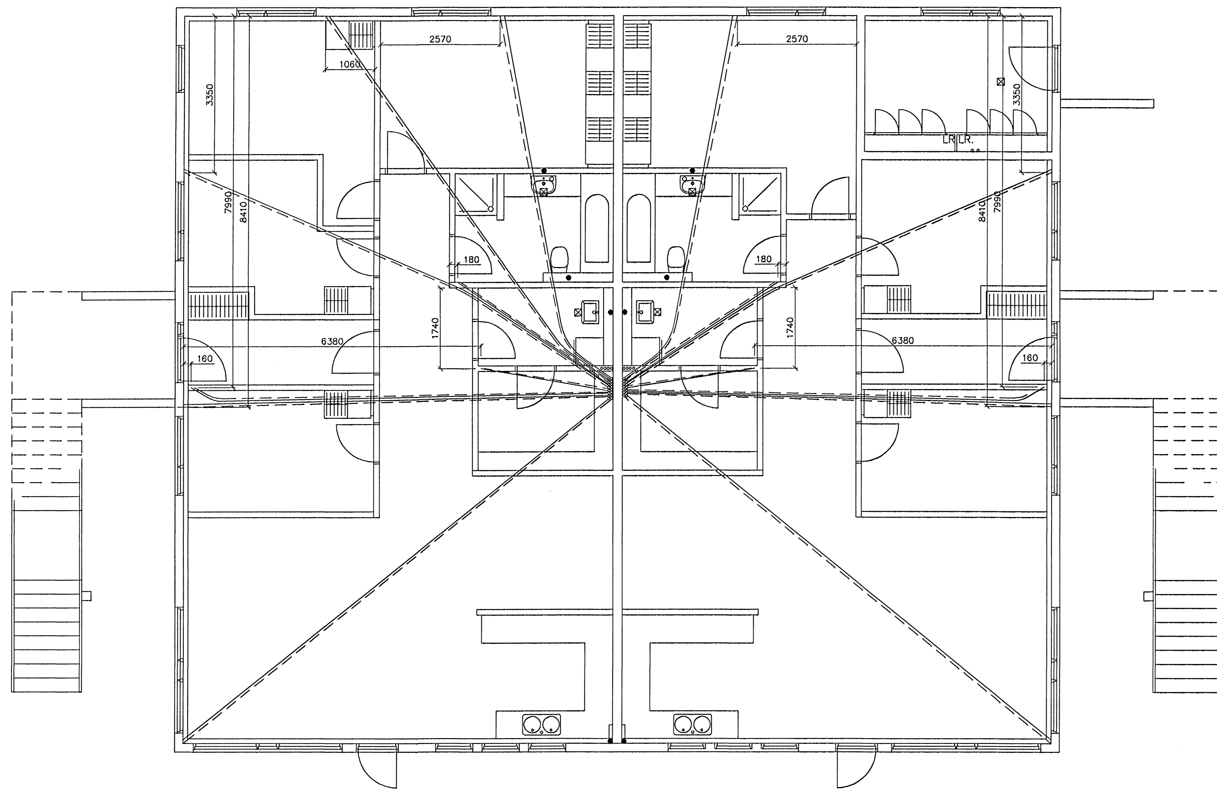
GRUNNMYND 1 HÆÐAR 1:50
