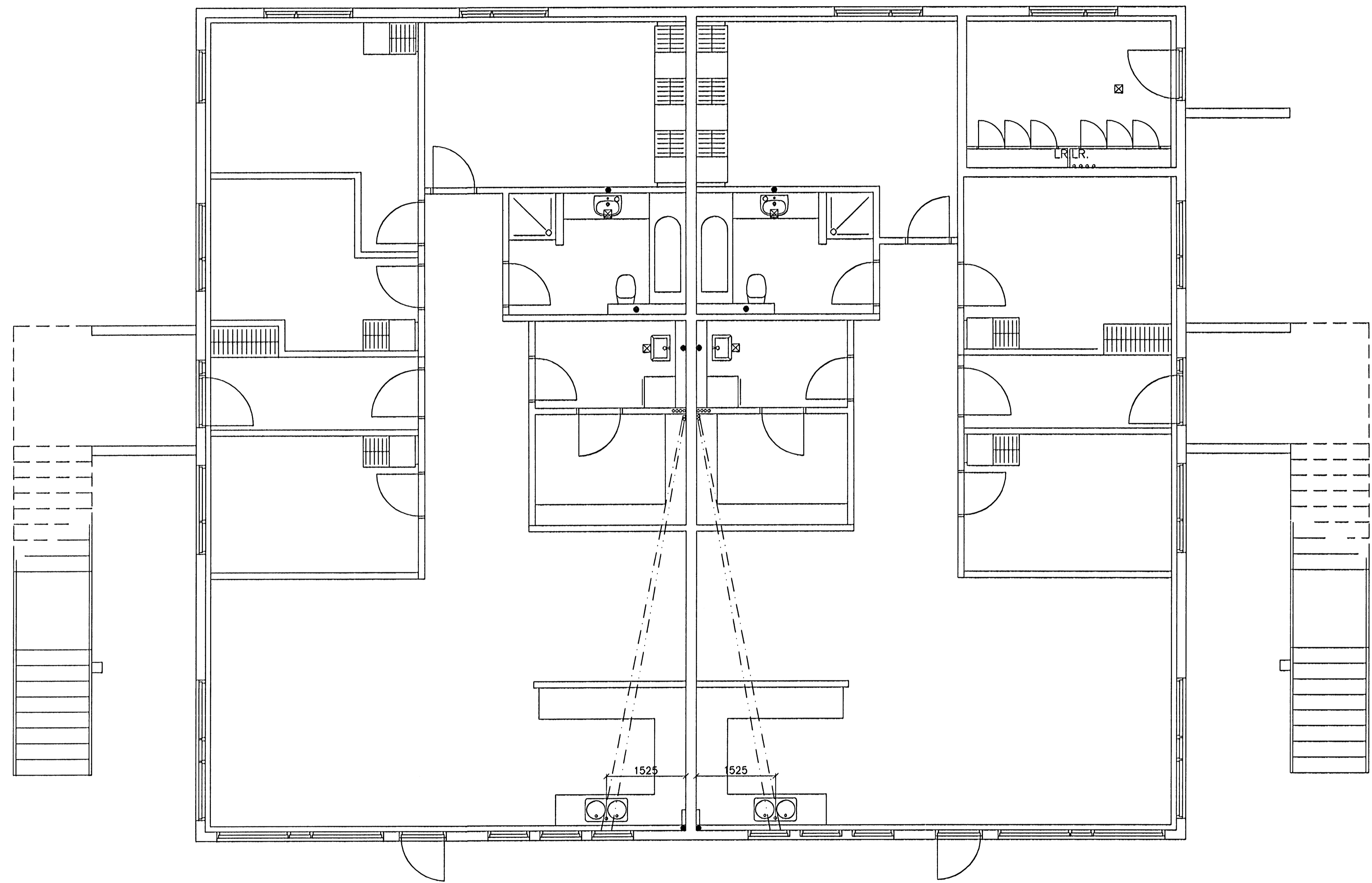
GRUNNMYND 1 HÆÐAR 1:50
