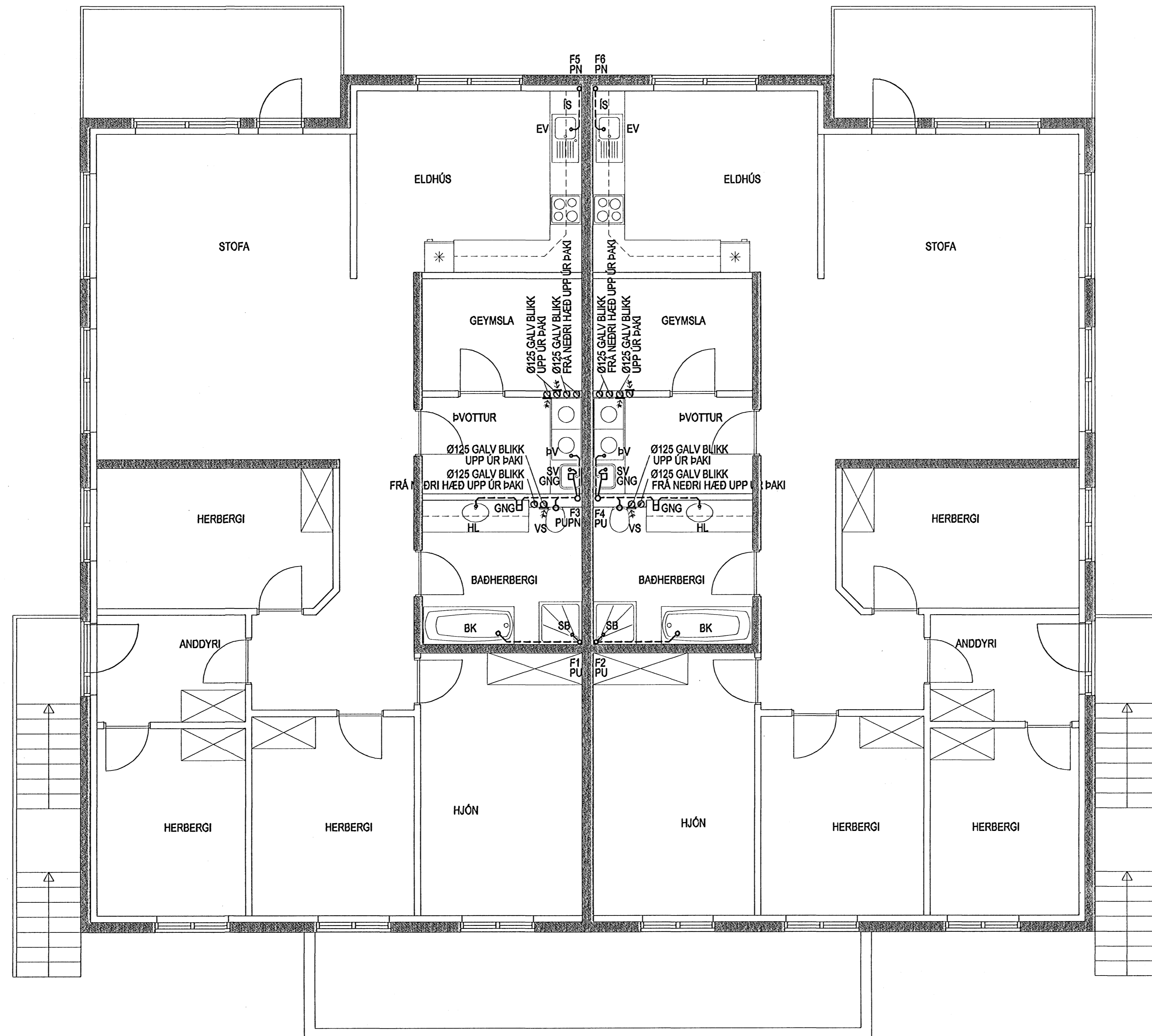
FRÁRENNISLAGNIR OG LOFTRÆSING GRUNNMYND EFRÍ HÆÐAR MKV. 1:50
