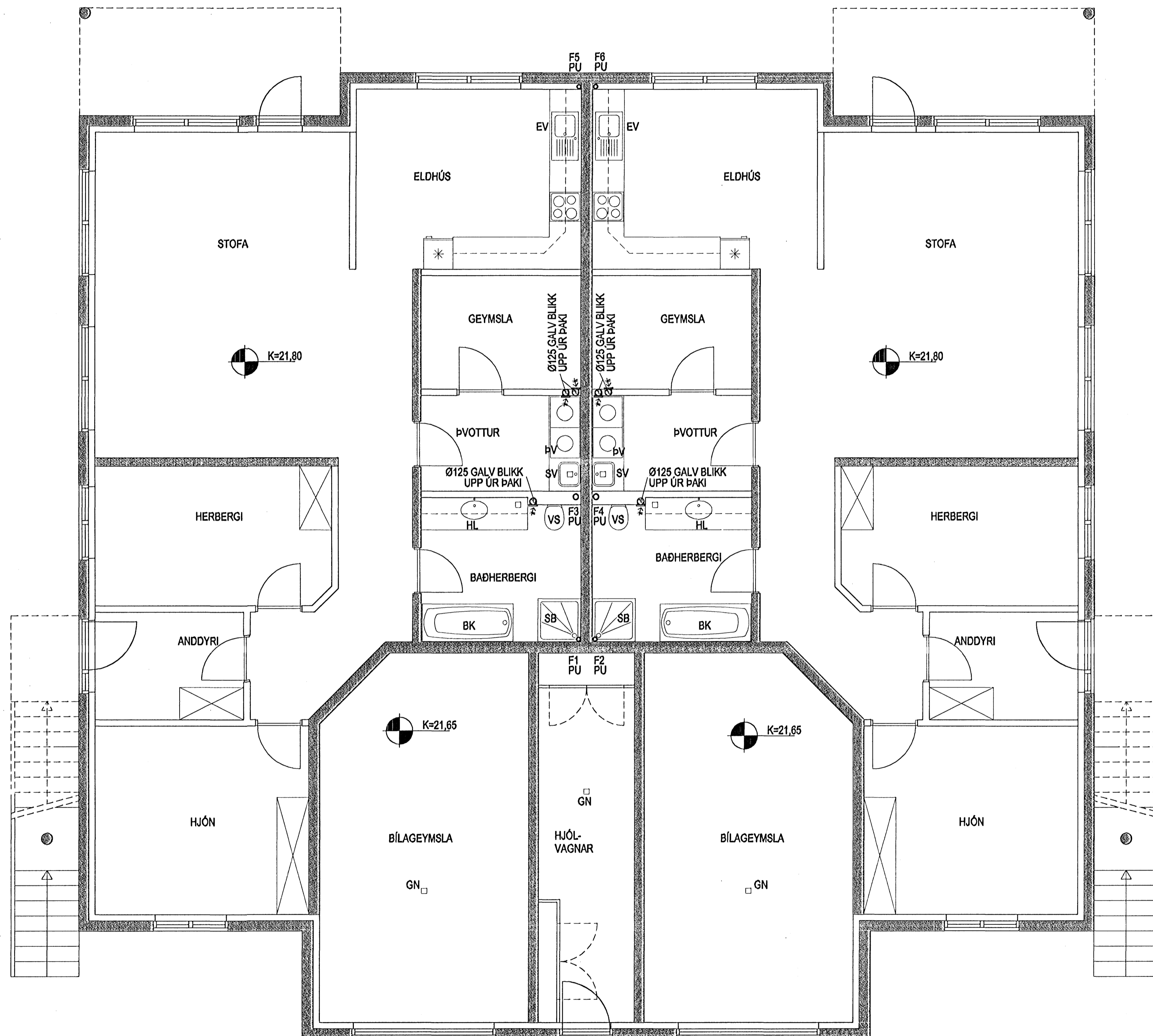
FRÁRENNSLISLAGNIR OG LOFTRÆSING GRUNNMYND NEDRI HÆÐAR MKV. 1:50
