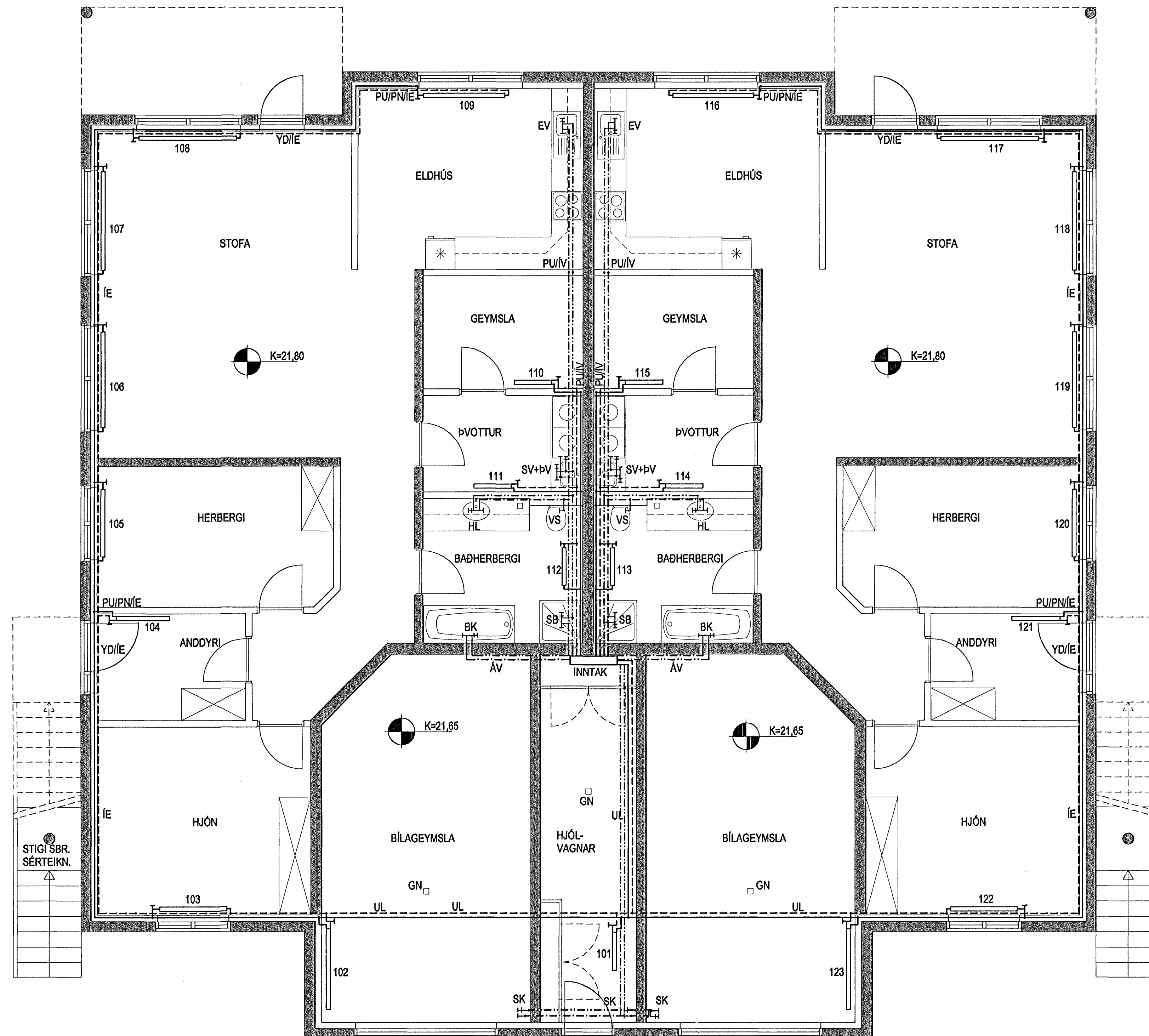
NEYSLUVATNS- OG HITALAGNIR GRUNNMYND NEDRI HÆÐAR MKV. 1:50
