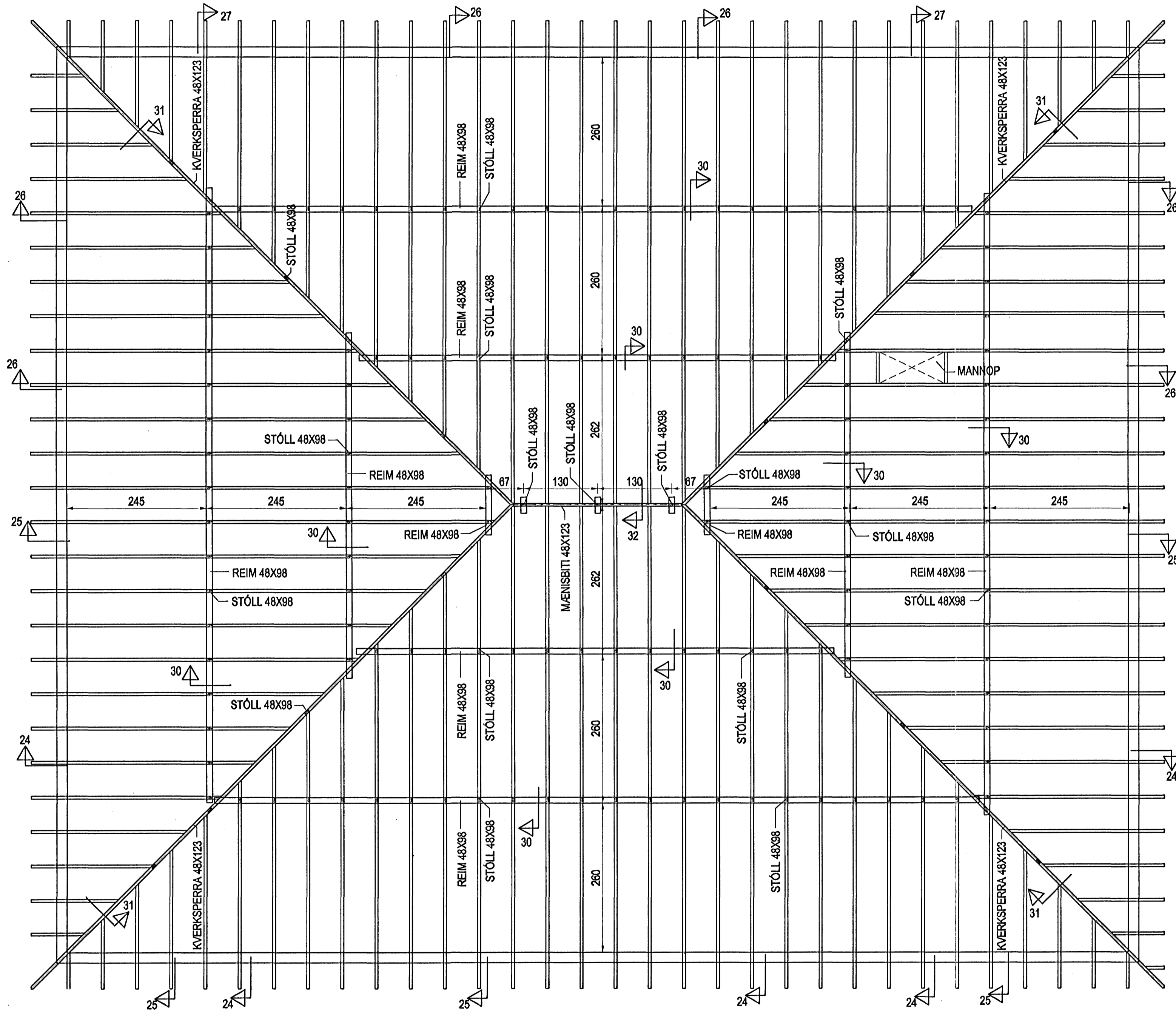
ÞAKVIÐIR, GRUNNMYND MKV. 1:50
