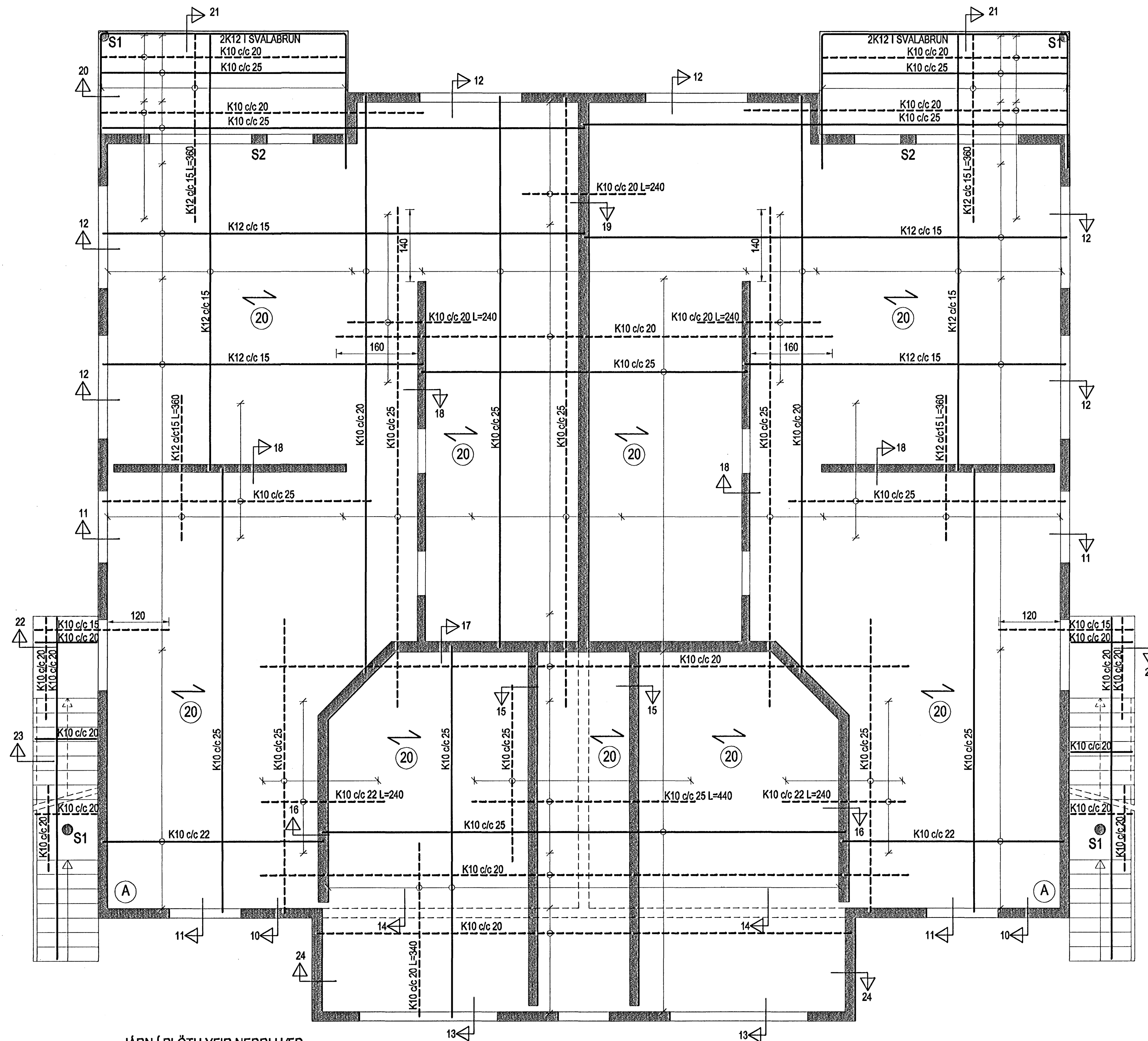
JÄRN Í PLÖTU YFIR NEDRI HÆÐ GRUNNMYND MKV. 1:50
