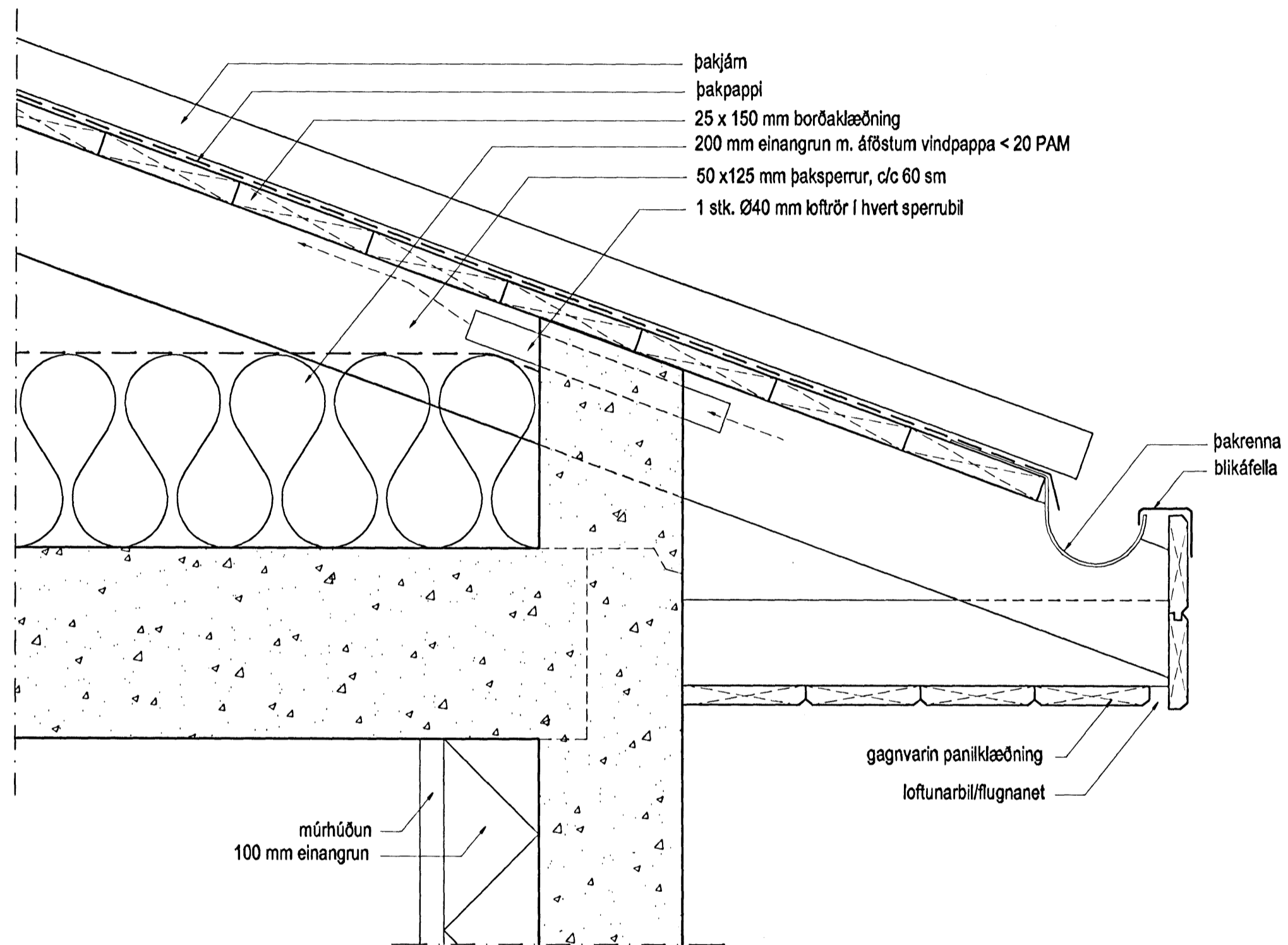
ÞAKBRÚN MKV. 1:5
