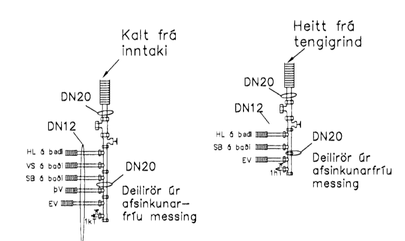
Deili – Tengimynd Málkvarði 1:20
