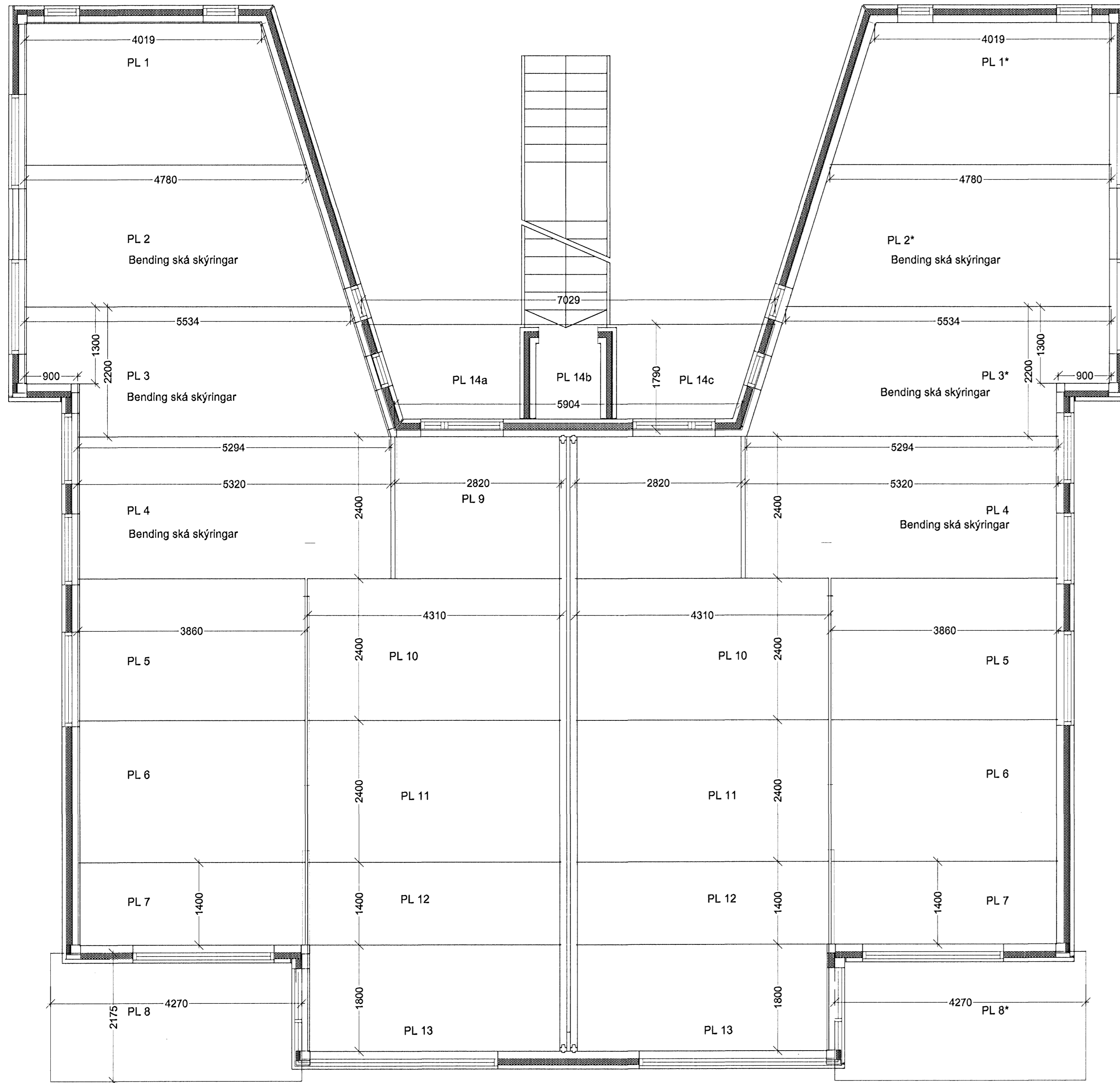
Filigranplötur grunnmynd 1 = 50 mm
