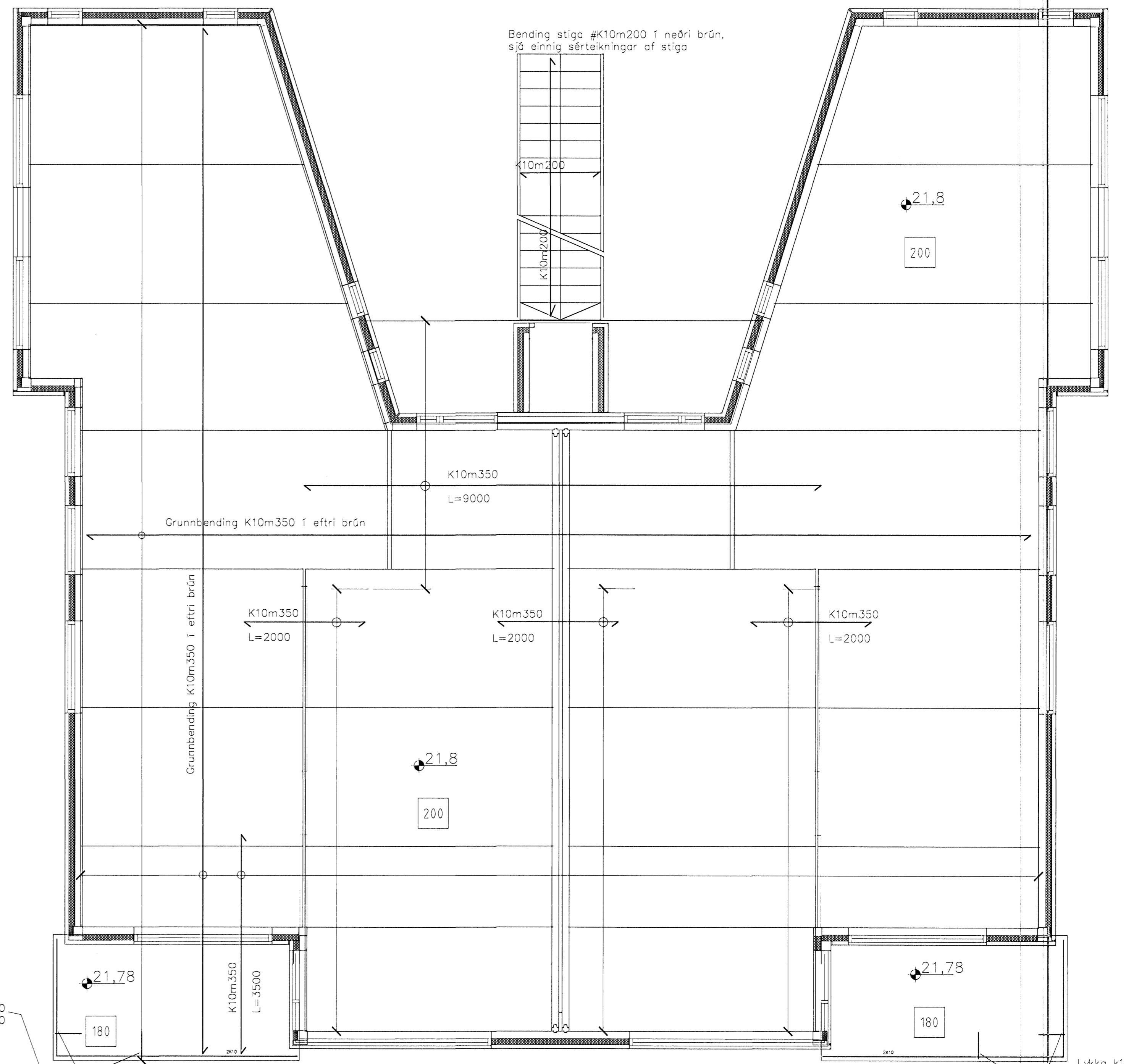
Járnbending plötu 2.hæð 1 = 50 mm
