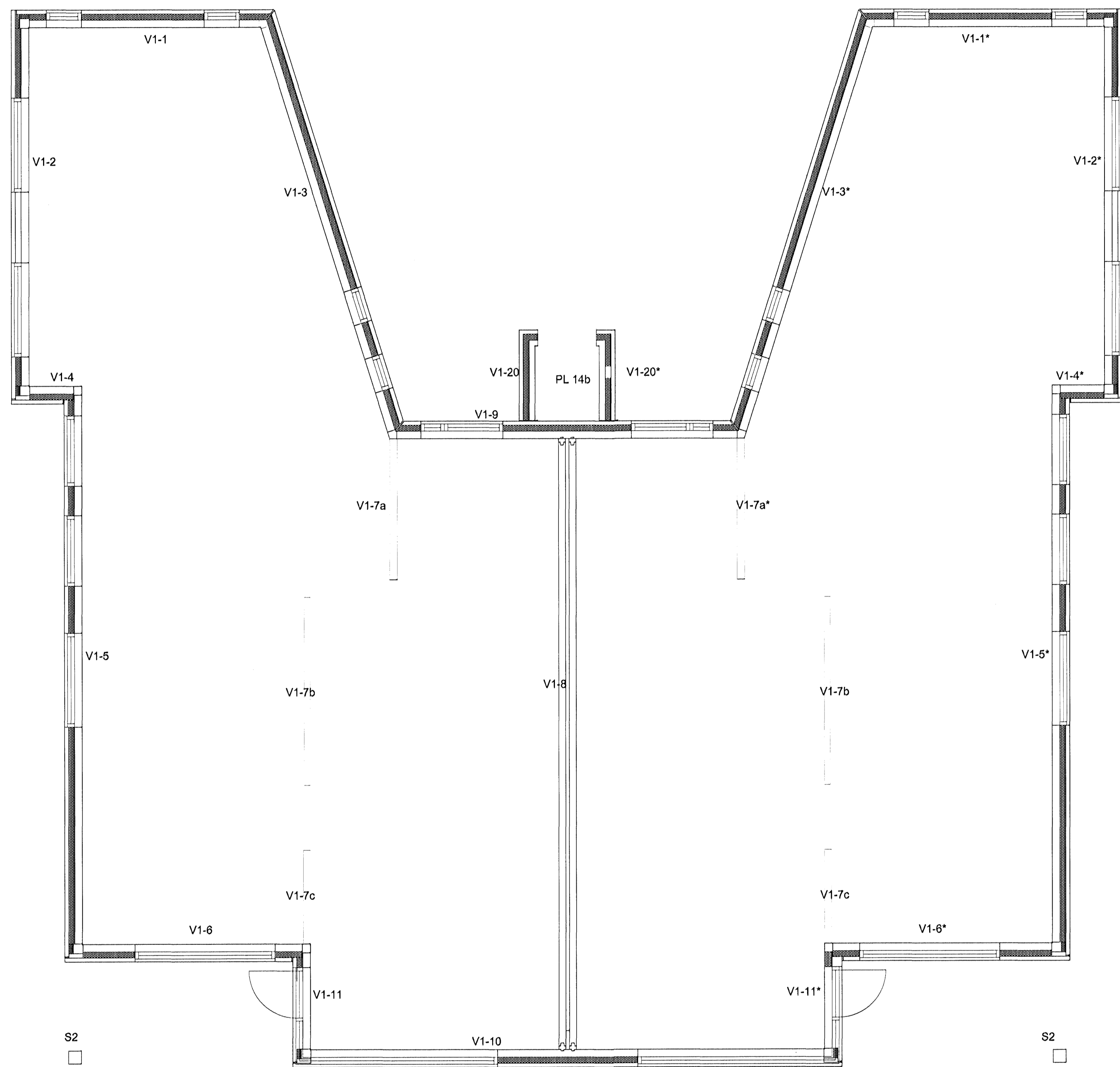
Veggeiningar 1.hæð grunnmynd 1 = 50 mm
